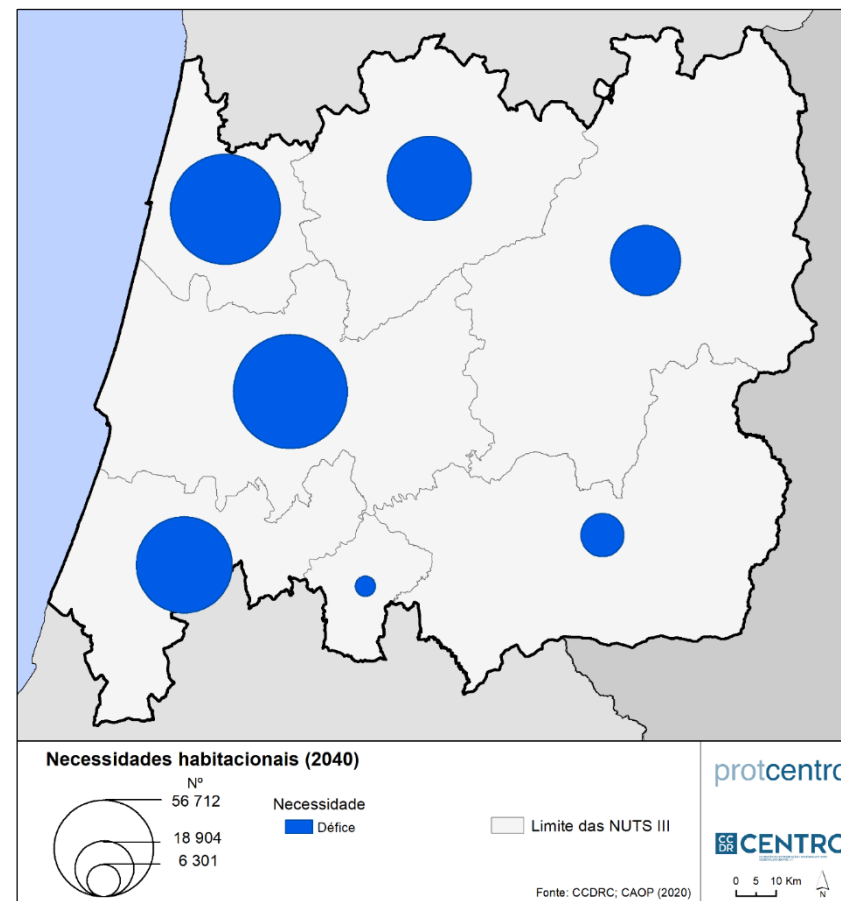
Figura 15. Necessidades habitacionais 2040
