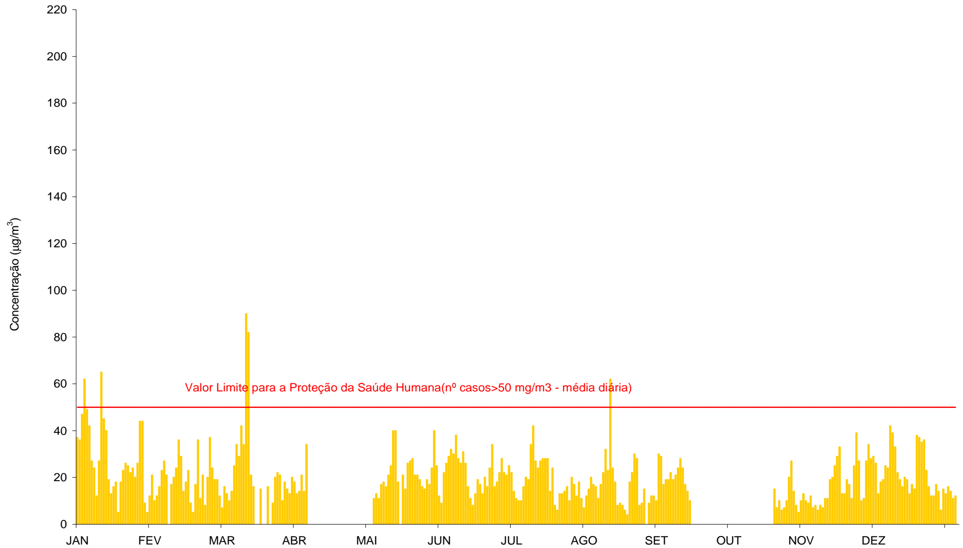
Gráfico 65 – Médias diárias das concentrações de PM10 ( \mu\text{g}/\text{m}^3 ) registadas em Coimbra/Instituto Geofísico (Janeiro a Dezembro de 2015).
