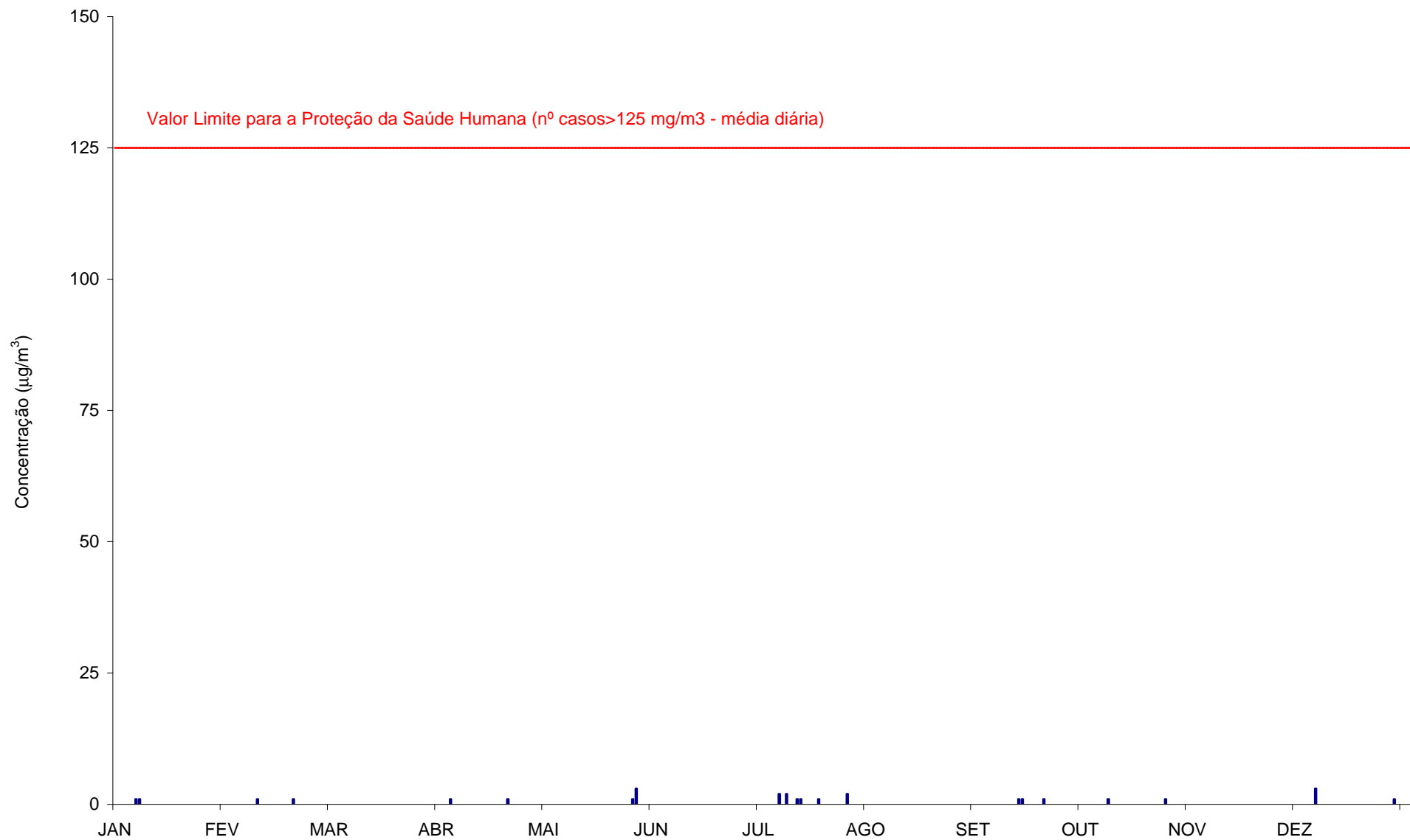
Gráfico 7 - Médias diárias das concentrações de \text{SO}_2 ( \mu\text{g}/\text{m}^3 ) registadas em Ílhavo (Janeiro a Dezembro de 2015).
