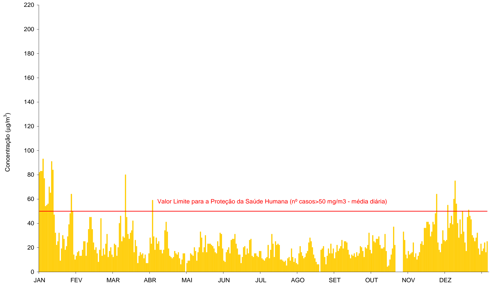
Gráfico 64 – Médias diárias das concentrações de PM10 ( \mu\text{g}/\text{m}^3 ) registadas em Aveiro (Janeiro a Dezembro de 2015).
