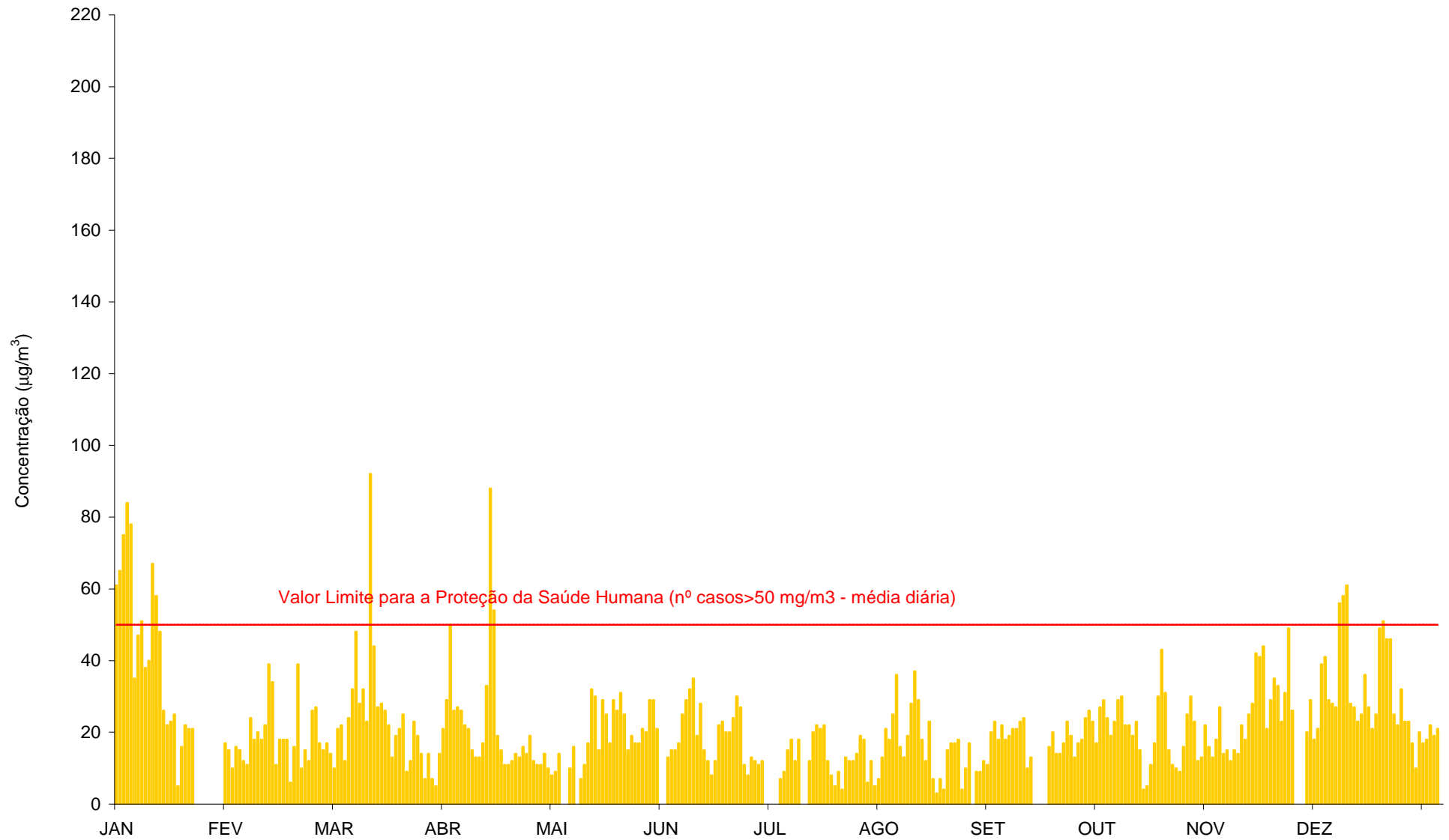
Gráfico 68 – Médias diárias das concentrações de PM10 ( \mu\text{g}/\text{m}^3 ) registadas na Ervedeira (Janeiro a Dezembro de 2015).
