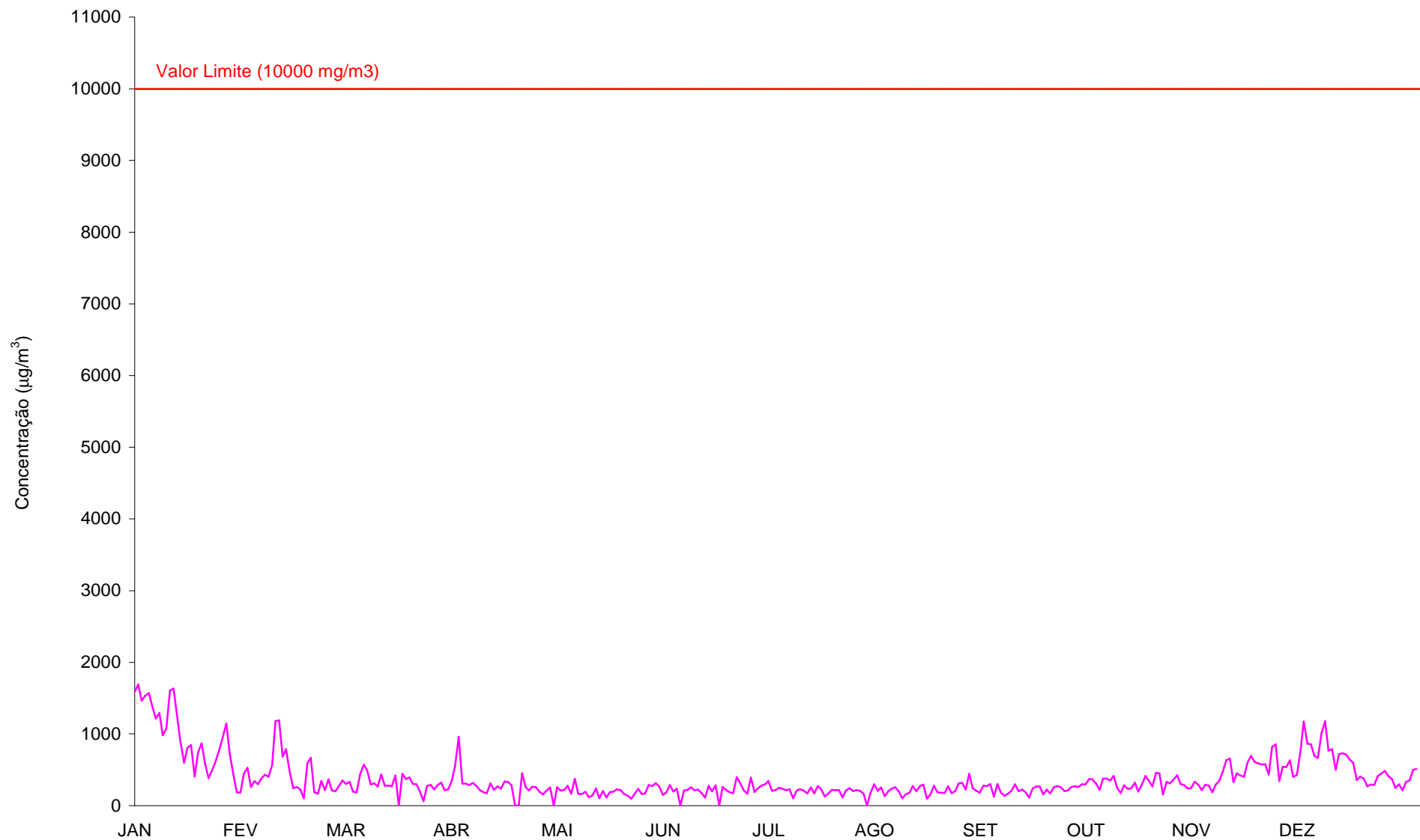
Gráfico 52 - Máximo diário das médias de oito horas das concentrações de CO ( \mu\text{g}/\text{m}^3 ) registadas em Aveiro (Janeiro a Dezembro de 2015).
