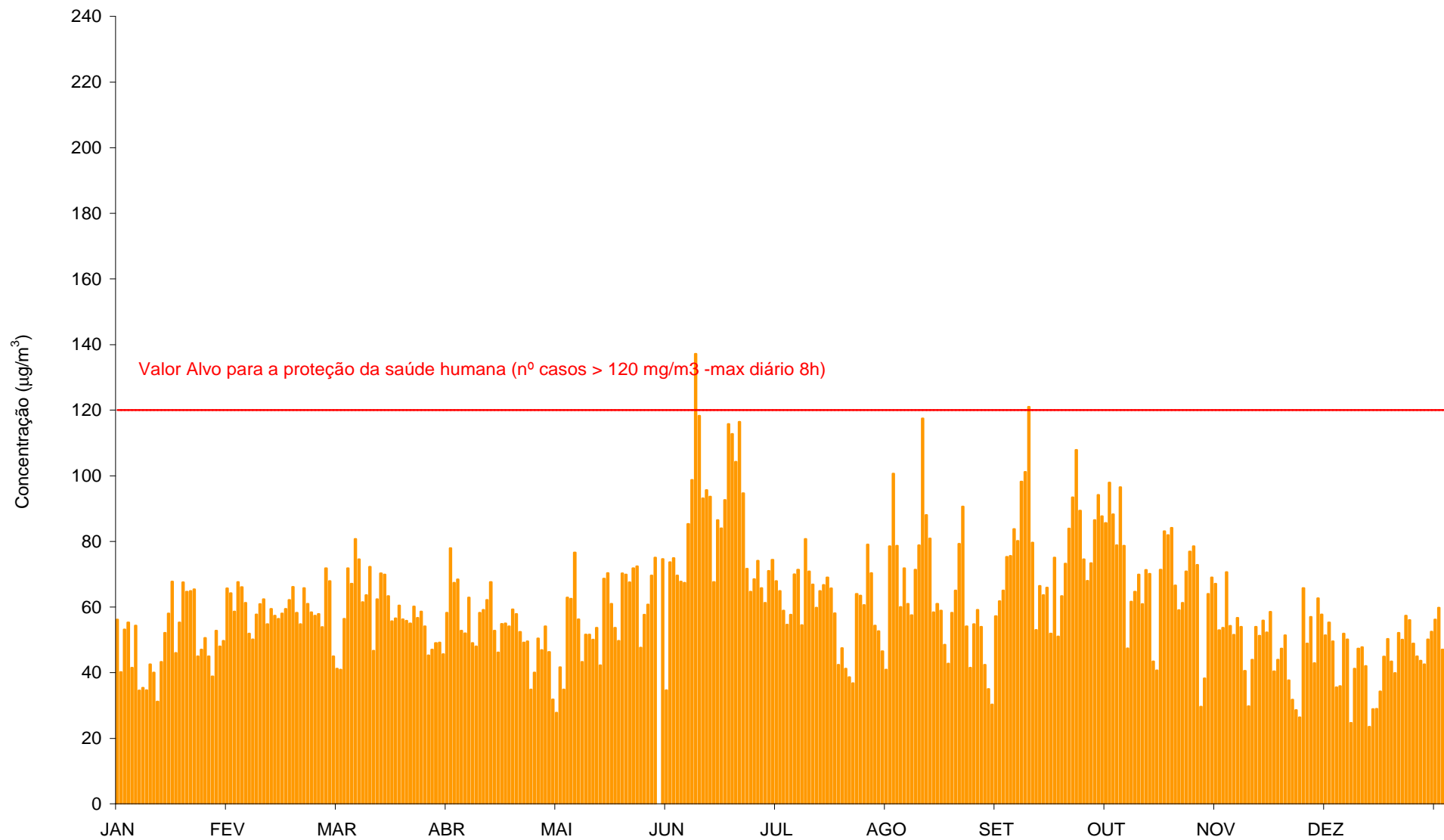
Gráfico 45 - Máximo das médias octo-horárias do dia das concentrações de O 3 ( \mu\text{g}/\text{m}^3 ) registadas em Ílhavo (Janeiro a Dezembro de 2015).
