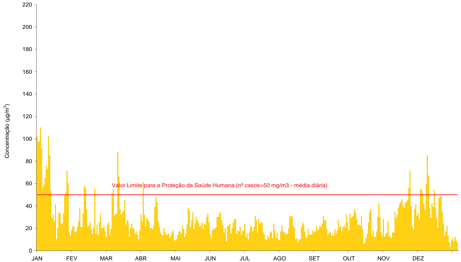
Gráfico 63 – Médias diárias das concentrações de PM10 ( \mu\text{g}/\text{m}^3 ) registadas em Ílhavo (Janeiro a Dezembro de 2015).
