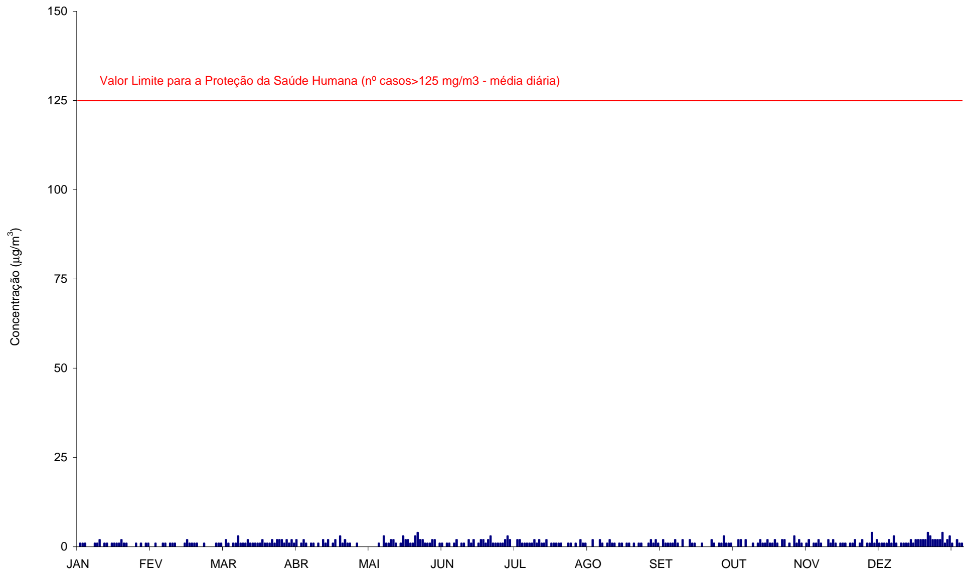
Gráfico 8 - Médias diárias das concentrações de \text{SO}_2 ( \mu\text{g}/\text{m}^3 ) registadas em Coimbra/Instituto Geofísico (Janeiro a Dezembro de 2015).
