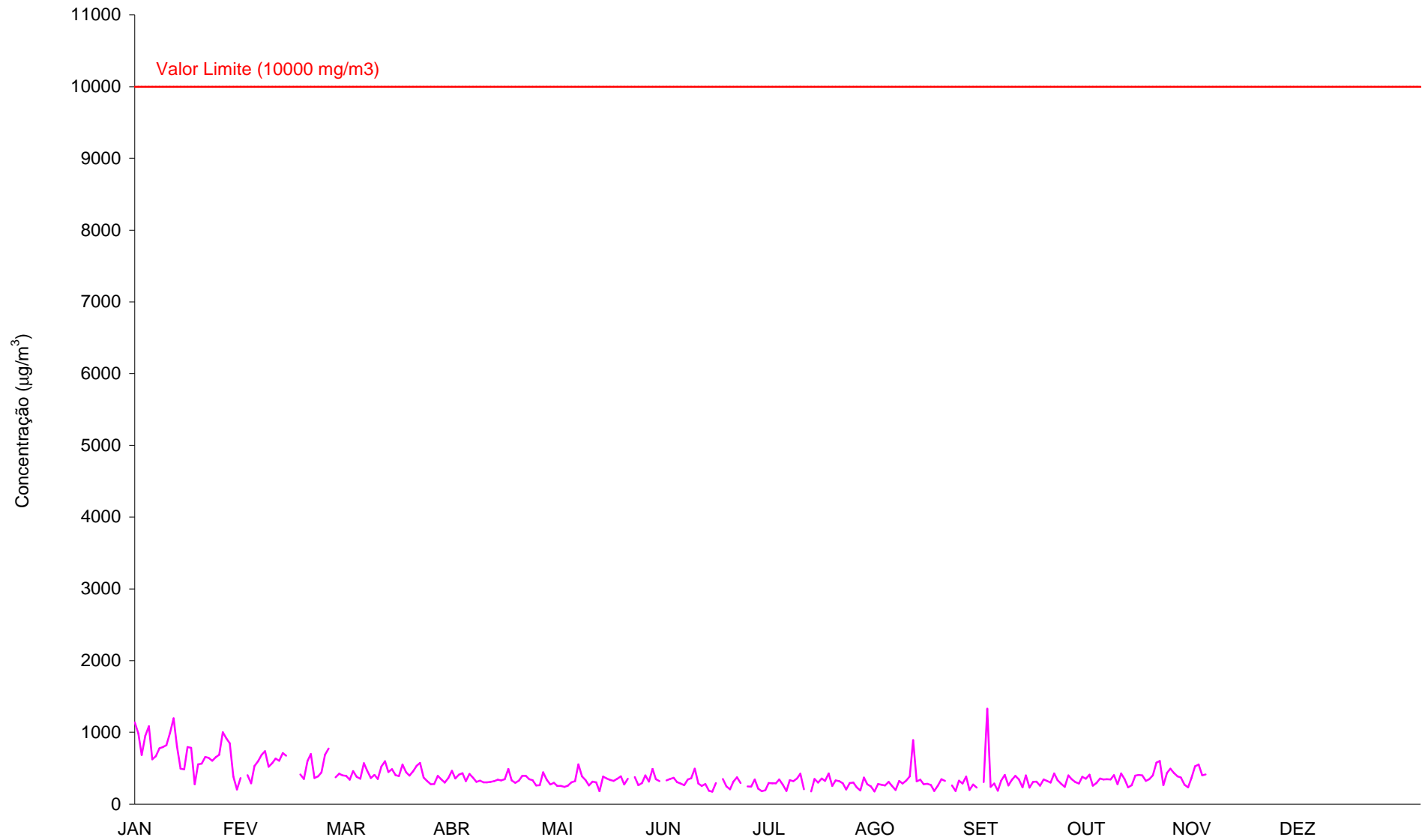
Gráfico 53 - Máximo diário das médias de oito horas das concentrações de CO ( \mu\text{g}/\text{m}^3 ) registadas em Coimbra/Fernão Magalhães (Janeiro a Dezembro de 2015).
