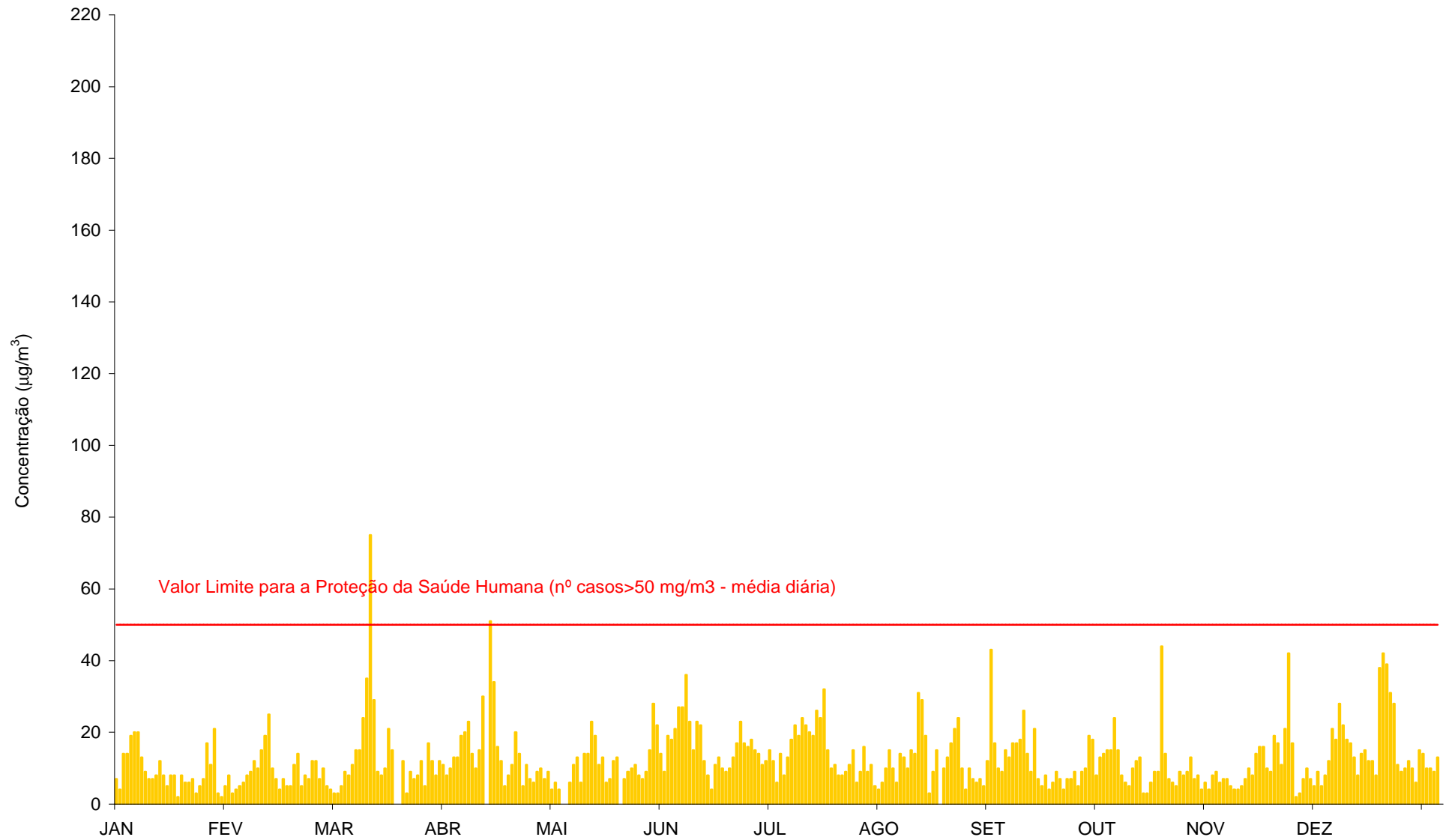
Gráfico 67 – Médias diárias das concentrações de PM10 ( \mu\text{g}/\text{m}^3 ) registadas em Furnelo do Monte (Janeiro a Dezembro de 2015).
