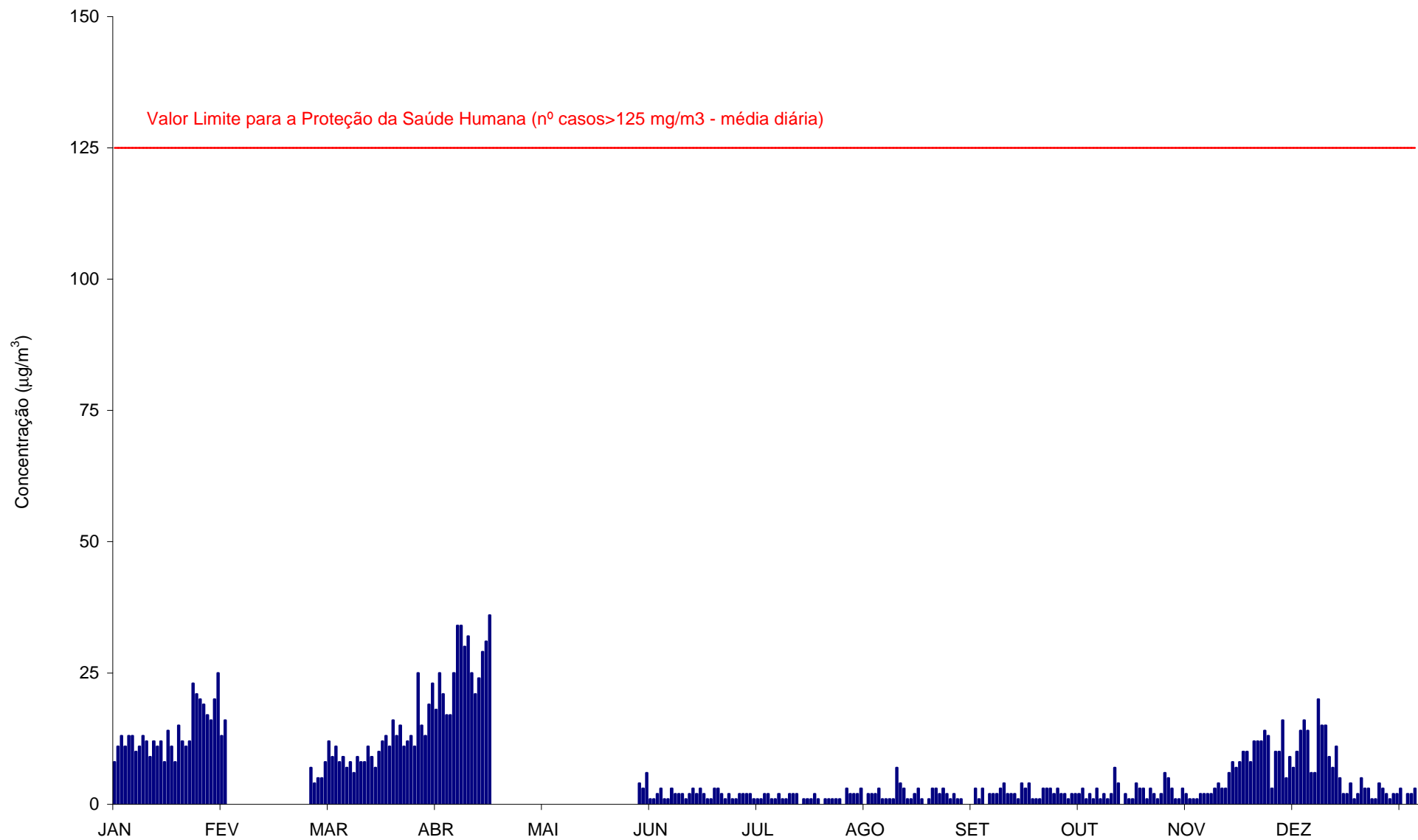
Gráfico 12 - Médias diárias das concentrações de \text{SO}_2 ( \mu\text{g}/\text{m}^3 ) registadas em Teixugueira (Janeiro a Dezembro de 2015).
