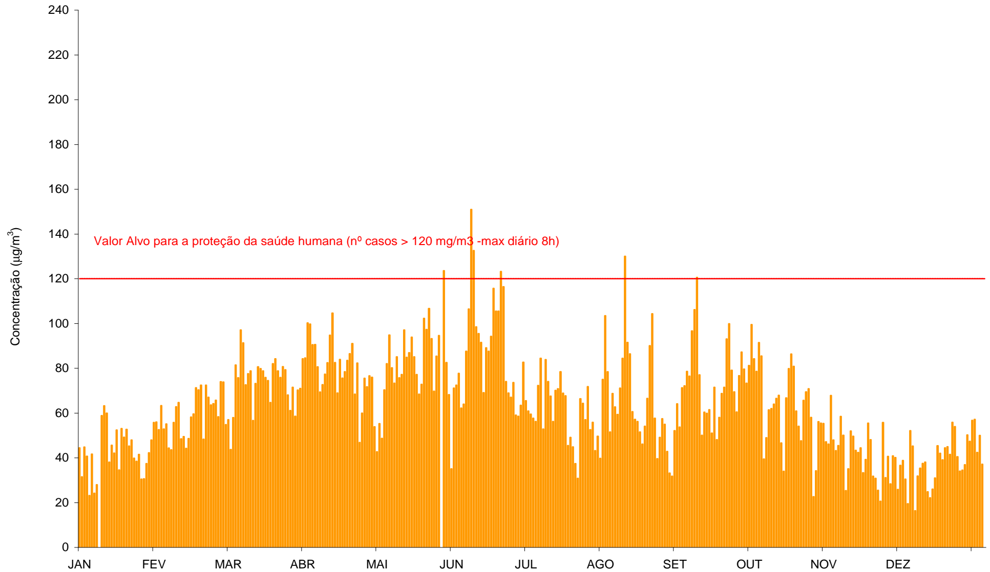
Gráfico 51 - Máximo das médias octo-horárias do dia das concentrações de O 3 ( \mu\text{g}/\text{m}^3 ) registadas na Teixugueira (Janeiro a Dezembro de 2015).
