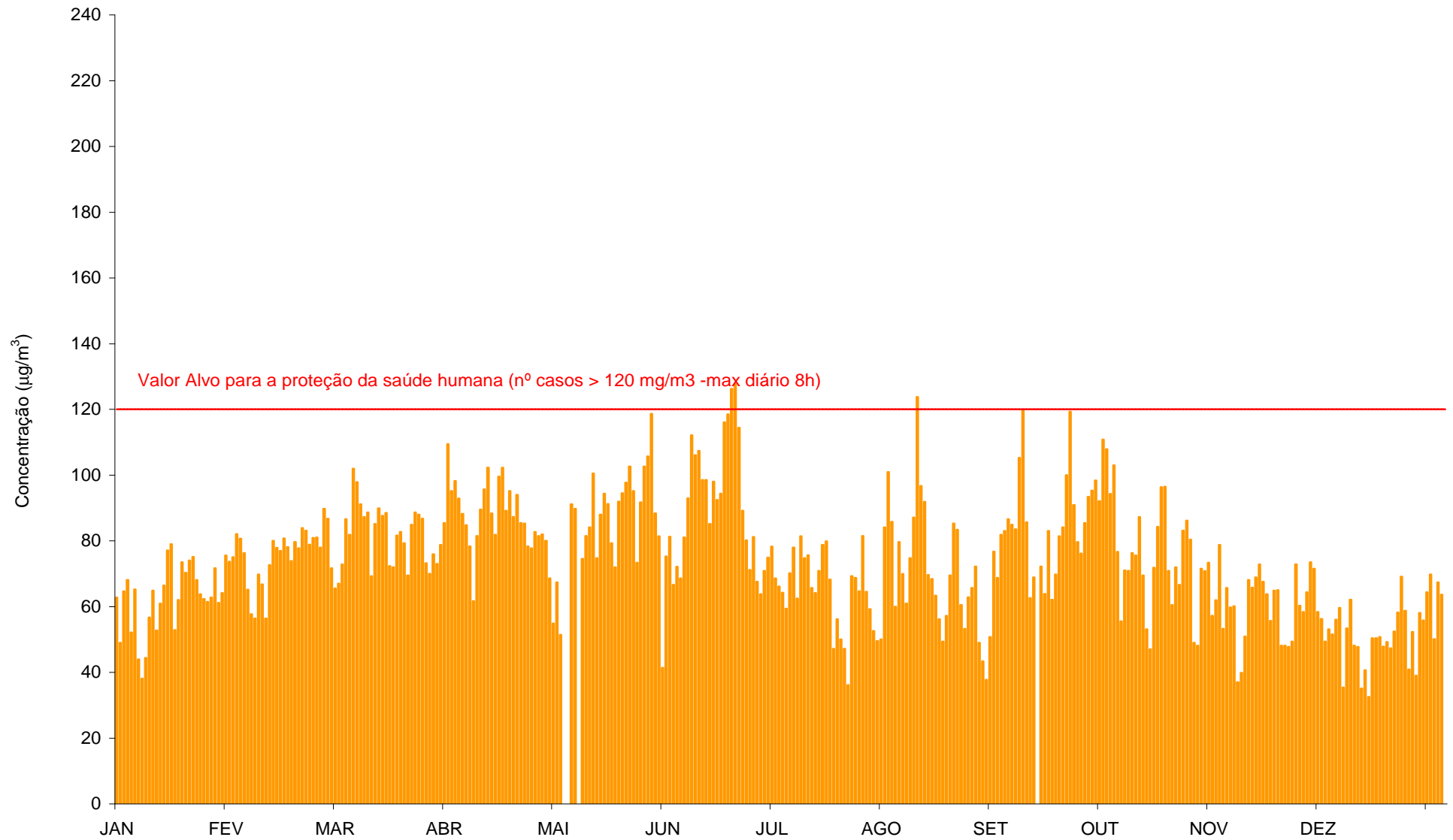
Gráfico 49 - Máximo das médias octo-horárias do dia das concentrações de O 3 ( \mu\text{g}/\text{m}^3 ) registadas em Ervedeira (Janeiro a Dezembro de 2015).
