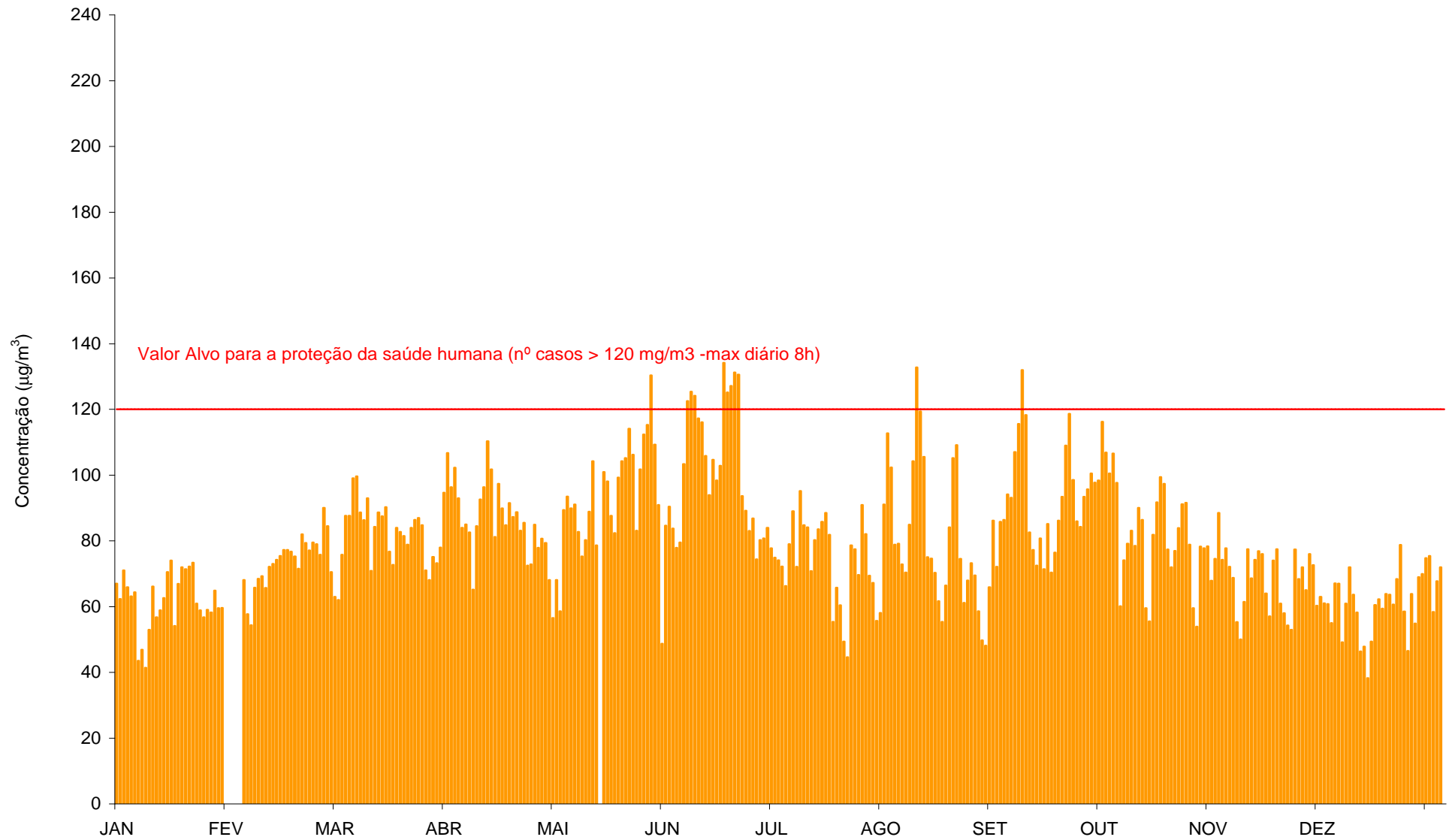
Gráfico 50 - Máximo das médias octo-horárias do dia das concentrações de O 3 ( \mu\text{g}/\text{m}^3 ) registadas em Montemor-o-Velho (Janeiro a Dezembro de 2015).
