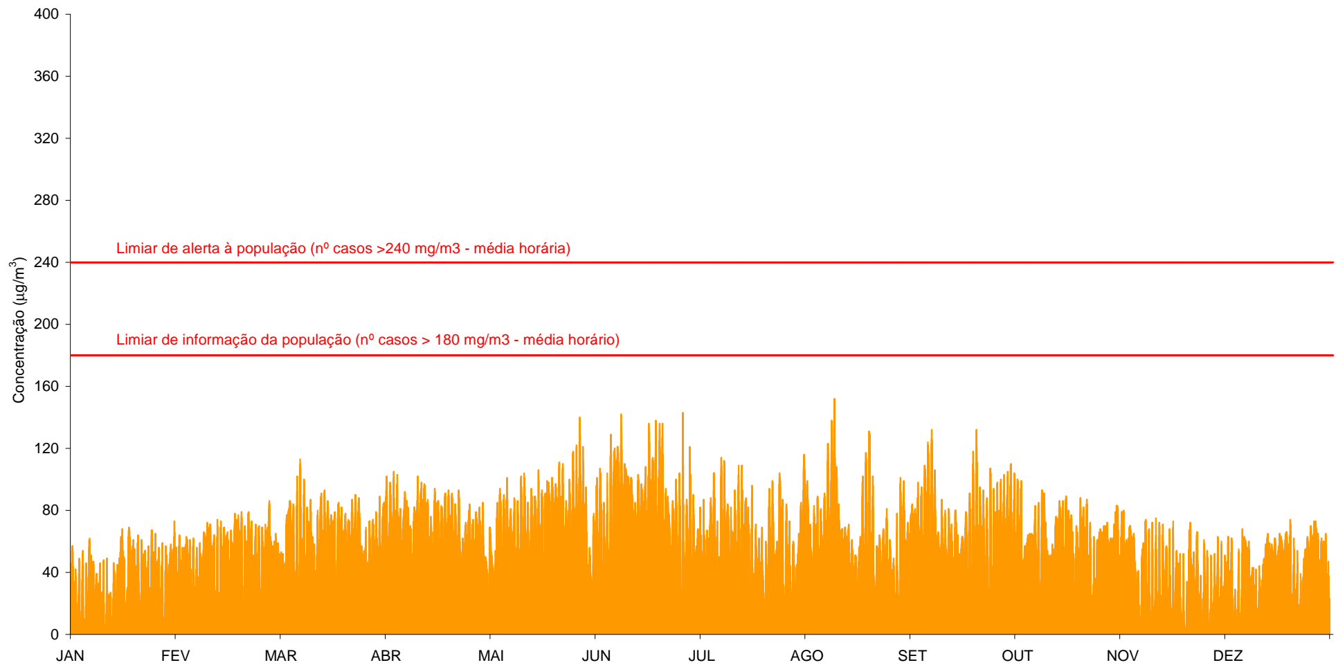
Gráfico 39 - Médias horárias das concentrações de O 3 (µg/m 3 ) registadas em Coimbra/Instituto Geofísico (Janeiro a Dezembro de 2015).
