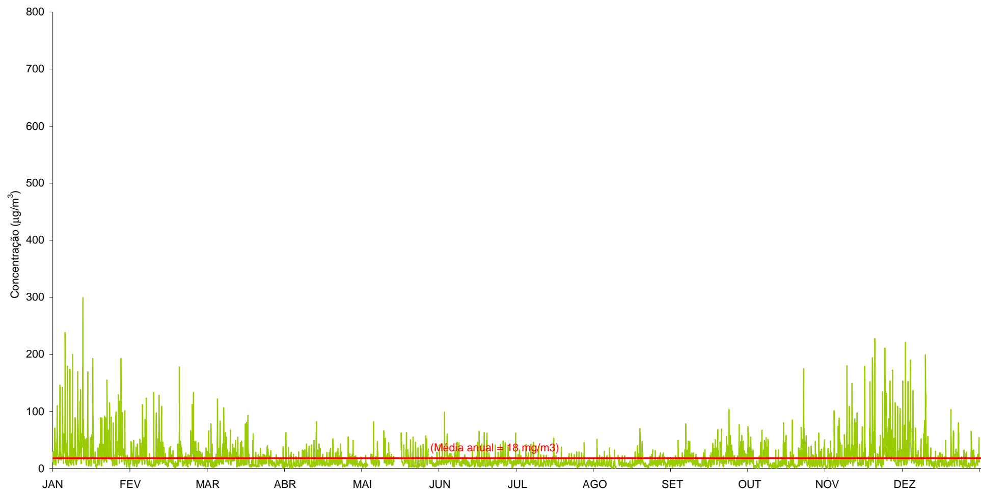
Gráfico 27 - Médias horárias das concentrações de \text{NO}_x ( \mu\text{g}/\text{m}^3 ) registadas em Coimbra/Instituto Geofísico (Janeiro a Dezembro de 2015).
