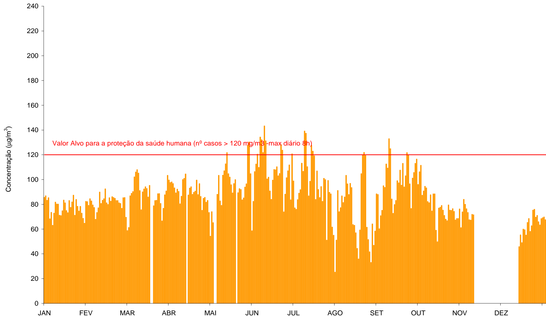
Gráfico 48 - Máximo das médias octo-horárias do dia das concentrações de \text{O}_3 ( \mu\text{g}/\text{m}^3 ) registadas em Furnel do Monte (Janeiro a Dezembro de 2015).
