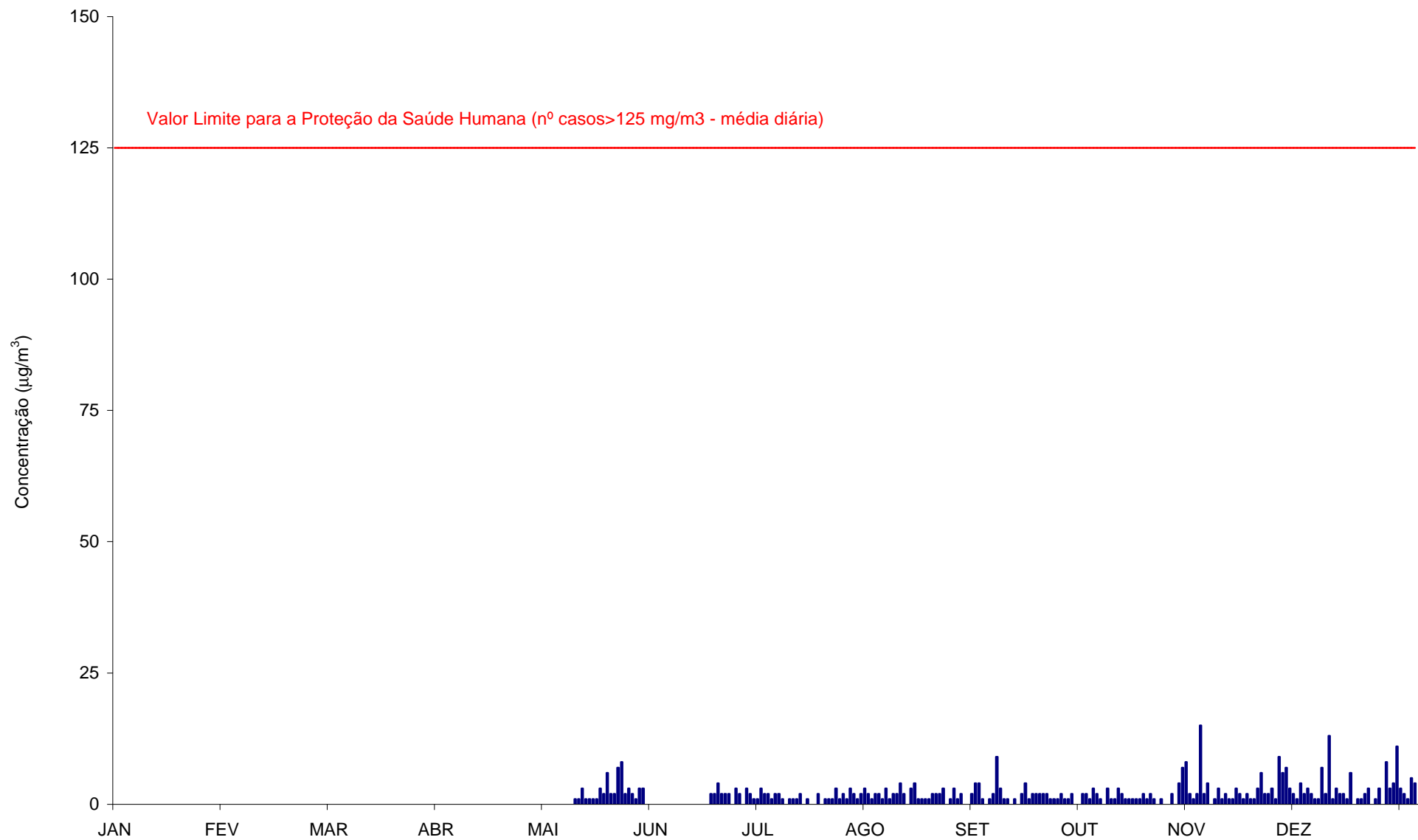
Gráfico 10 - Médias diárias das concentrações de \text{SO}_2 ( \mu\text{g}/\text{m}^3 ) registadas em Ervedeira (Janeiro a Dezembro de 2015).
