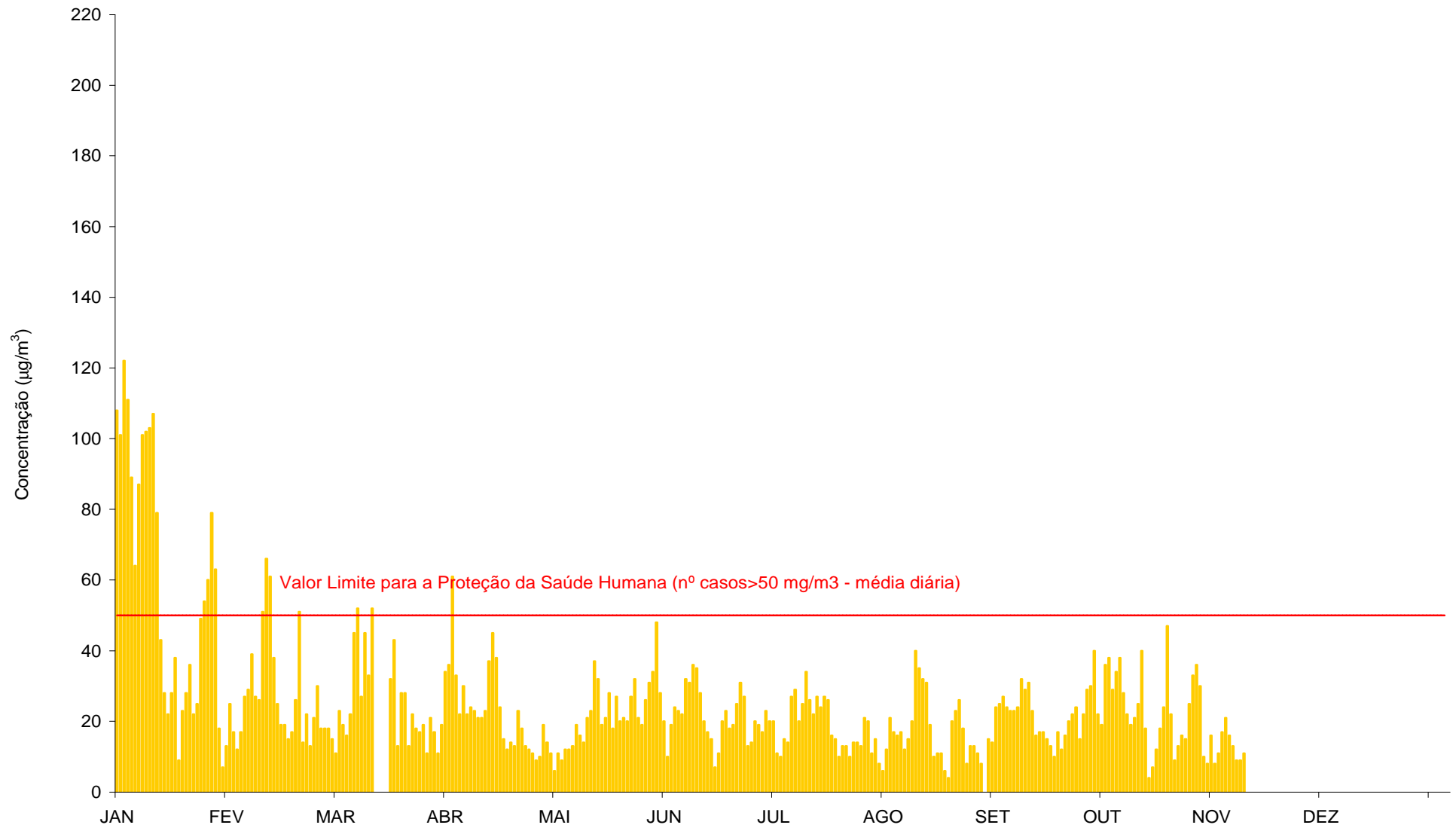
Gráfico 71 – Médias diárias das concentrações de PM10 ( \mu\text{g}/\text{m}^3 ) registadas na Teixugueira (Janeiro a Dezembro de 2015).
