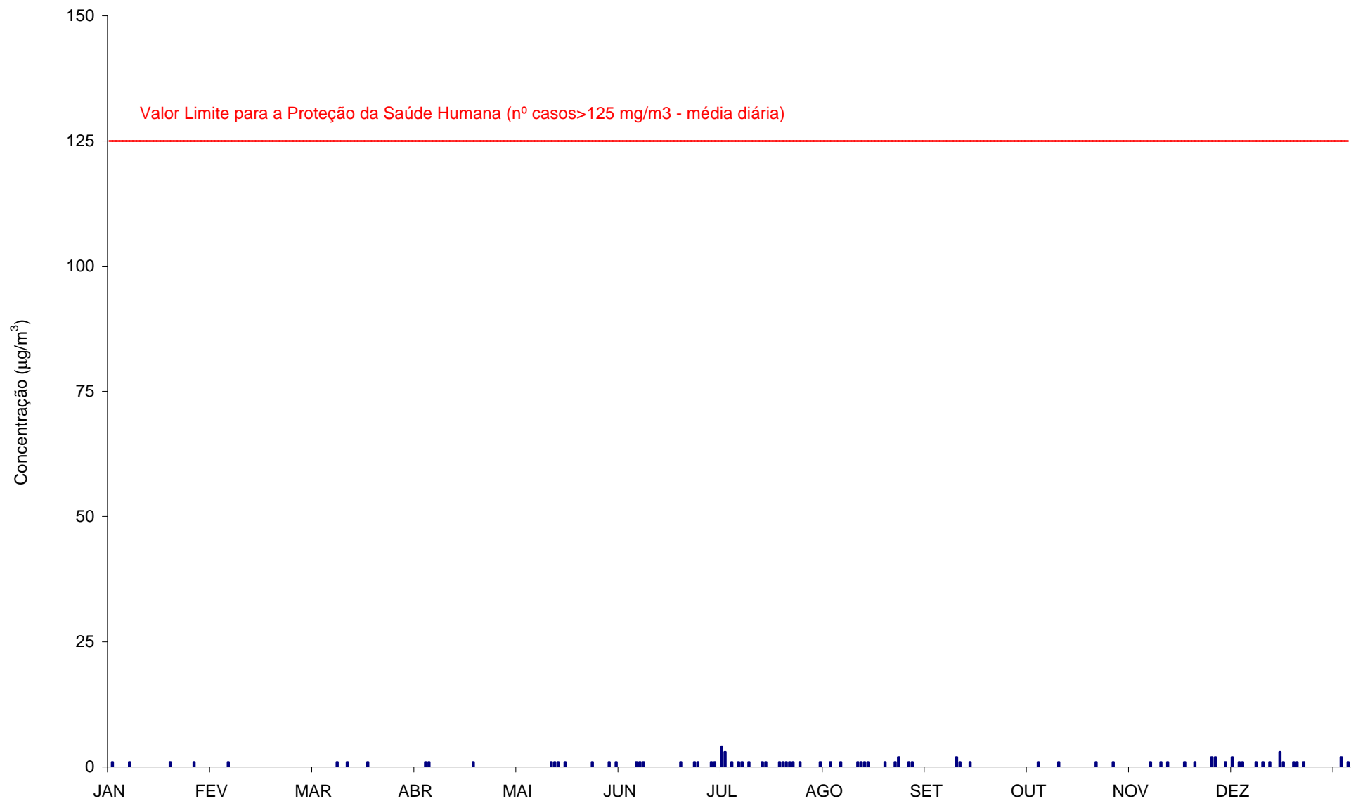
Gráfico 9 - Médias diárias das concentrações de \text{SO}_2 ( \mu\text{g}/\text{m}^3 ) registadas em Salgueiro (Janeiro a Dezembro de 2015).
