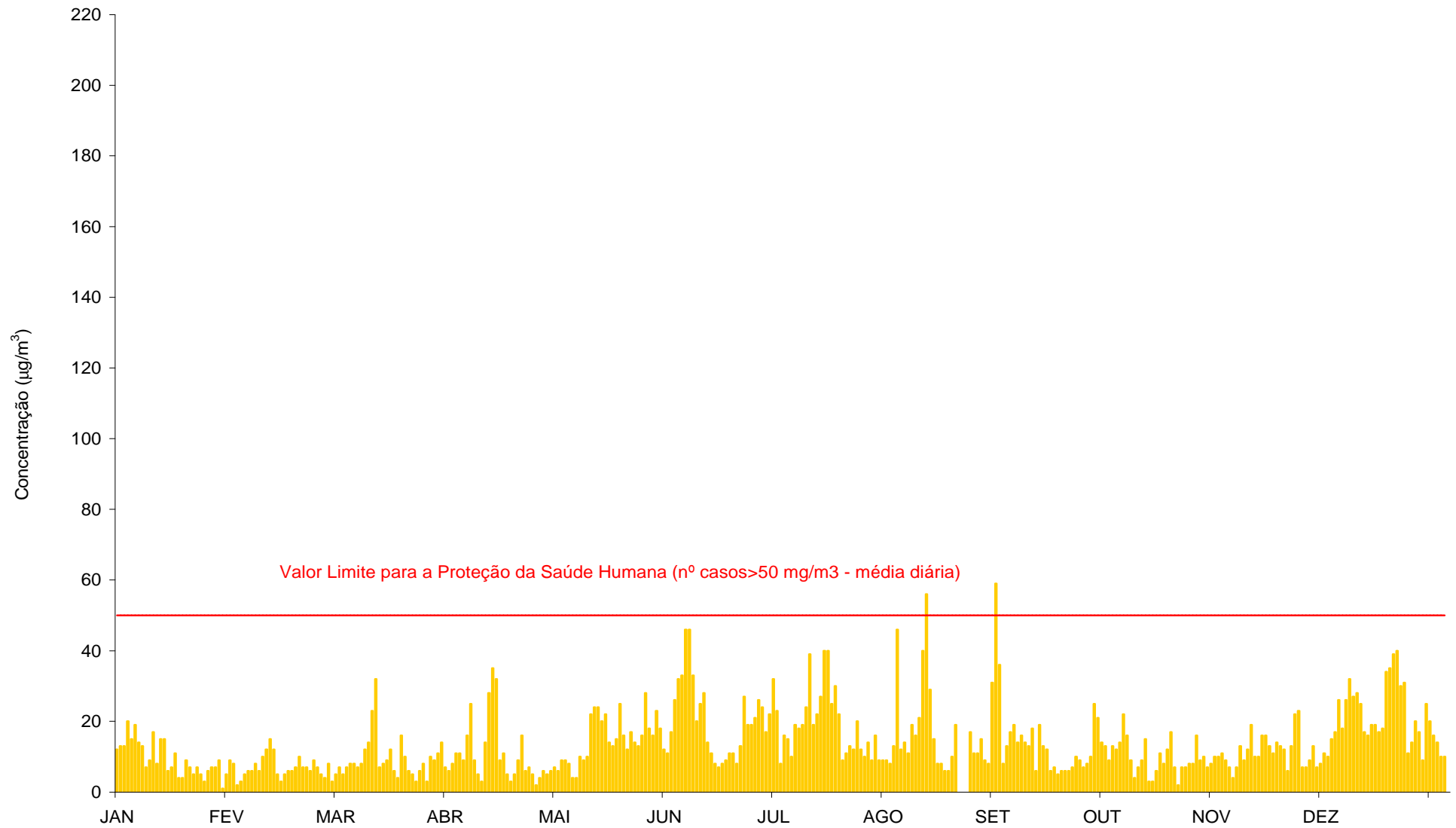
Gráfico 66 – Médias diárias das concentrações de PM 10 ( \mu\text{g}/\text{m}^3 ) registadas em Salgueiro (Janeiro a Dezembro de 2015).
