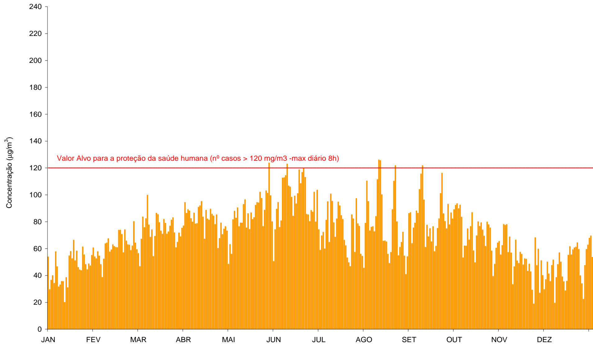
Gráfico 47 - Máximo das médias octo-horárias do dia das concentrações de \text{O}_3 ( \mu\text{g}/\text{m}^3 ) registadas em Salgueiro (Janeiro a Dezembro de 2015).
