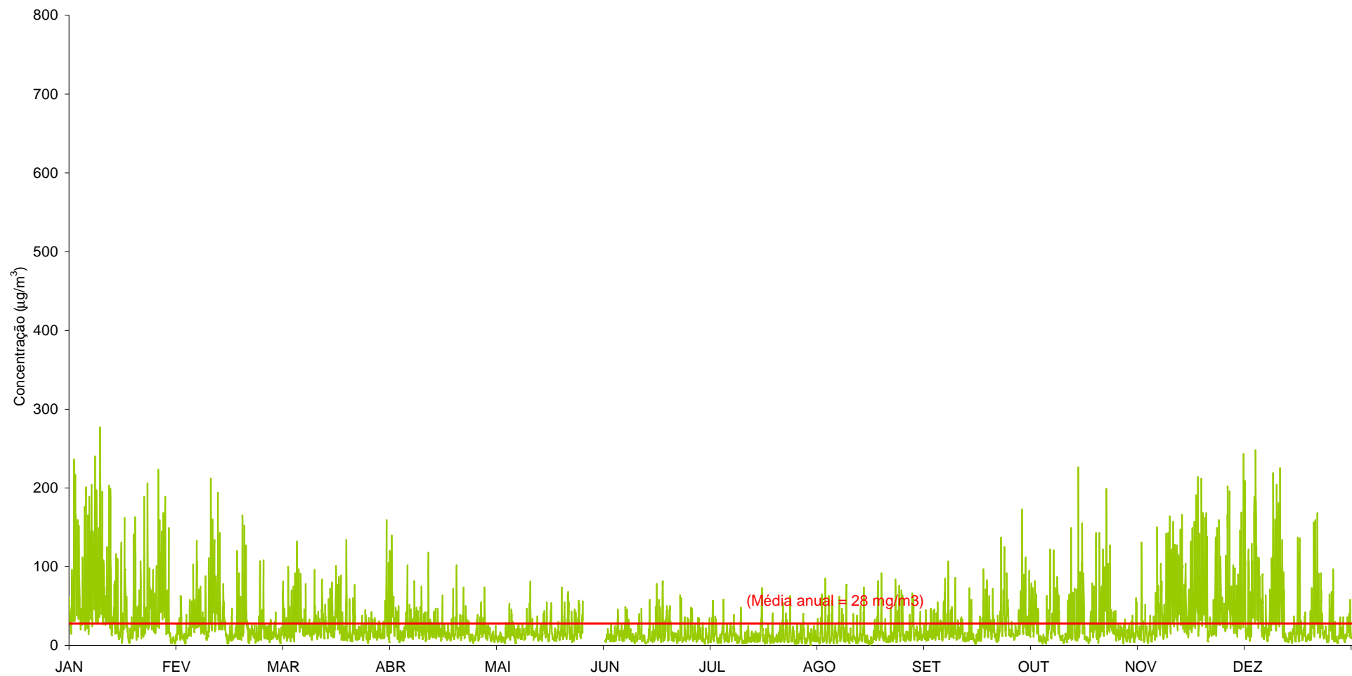
Gráfico 33 - Médias horárias das concentrações de \text{NO}_x ( \mu\text{g}/\text{m}^3 ) registadas na Teixugueira (Janeiro a Dezembro de 2015).
