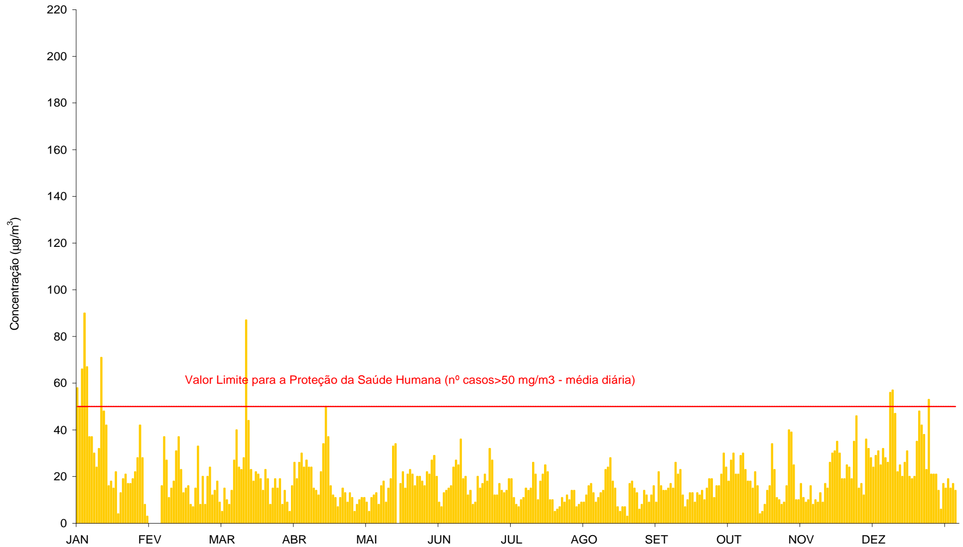
Gráfico 70 – Médias diárias das concentrações de PM10 ( \mu\text{g}/\text{m}^3 ) registadas em Montemor-o-Velho (Janeiro a Dezembro de 2015).
