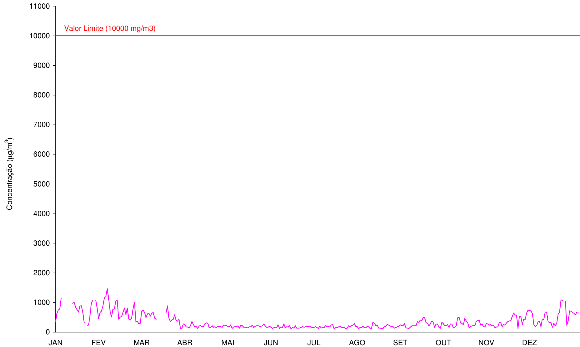
Gráfico 55 - Máximo diário das médias de oito horas das concentrações de CO ( \mu\text{g}/\text{m}^3 ) registadas em Aveiro (Janeiro a Dezembro de 2011).
