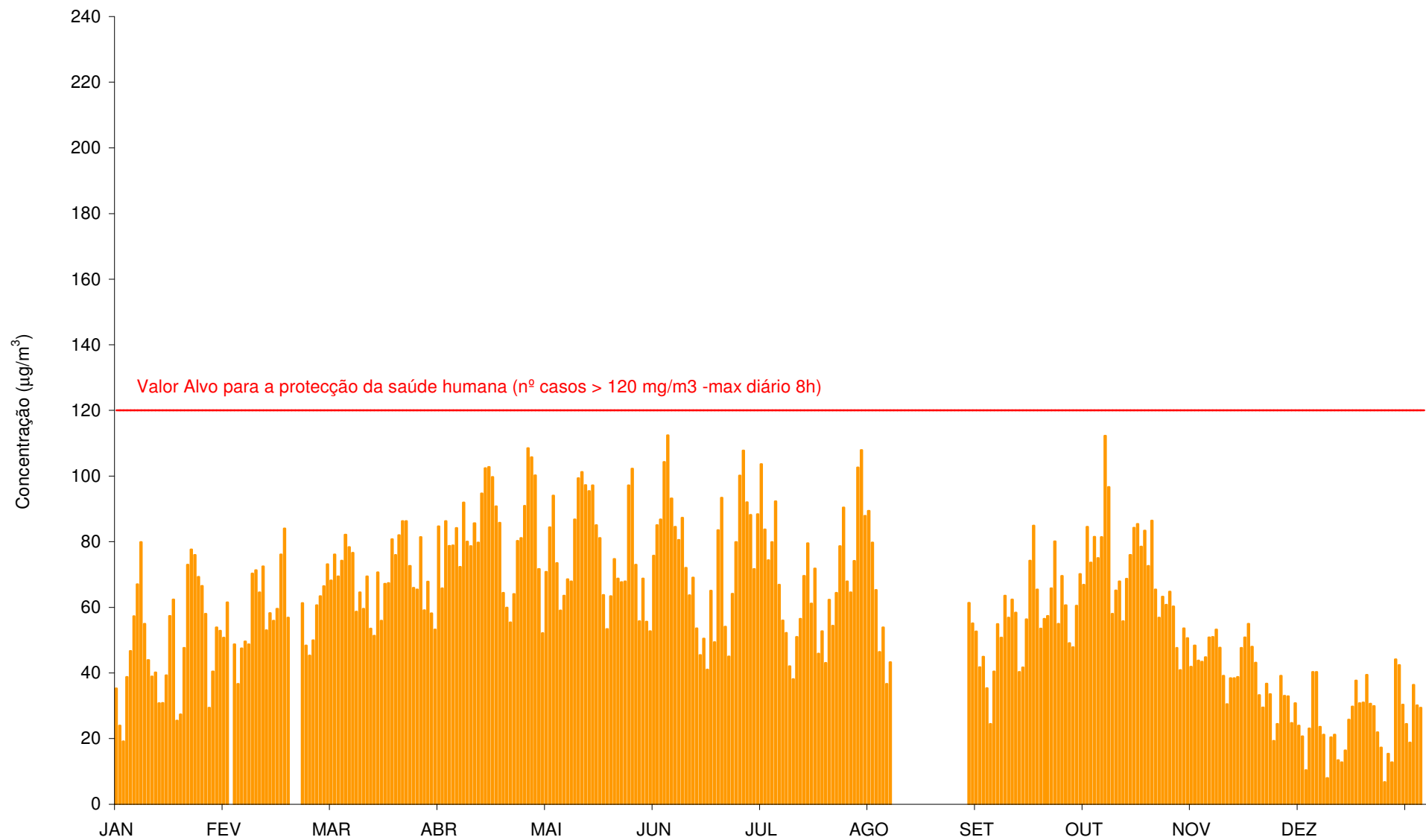
Gráfico 49 - Máximo das médias octo-horárias do dia das concentrações de \text{O}_3 ( \mu\text{g}/\text{m}^3 ) registadas no Instituto Geofísico (Janeiro a Dezembro de 2011).
