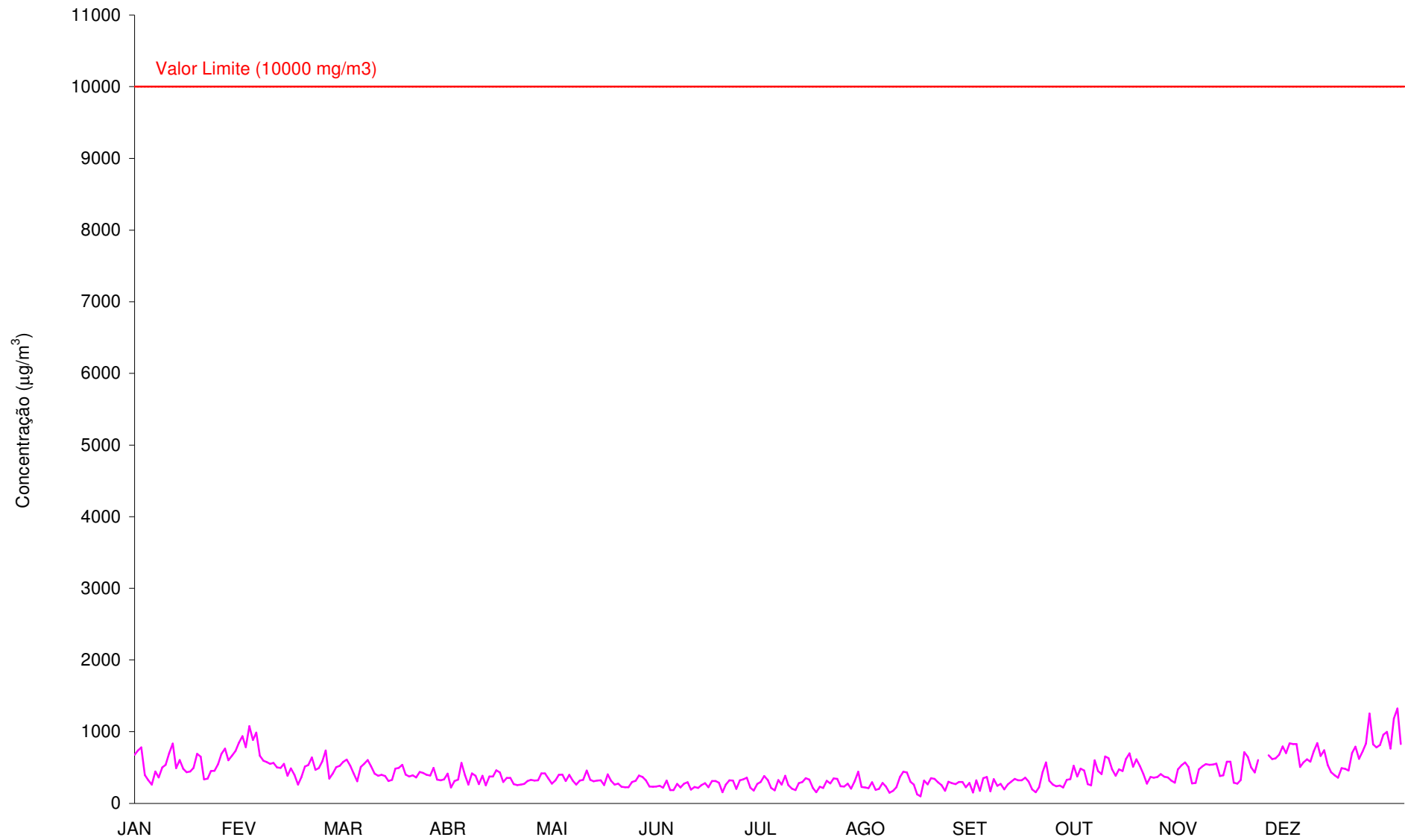
Gráfico 56 - Máximo diário das médias de oito horas das concentrações de CO ( \mu\text{g}/\text{m}^3 ) registadas na Fernão Magalhães (Janeiro a Dezembro de 2011).
