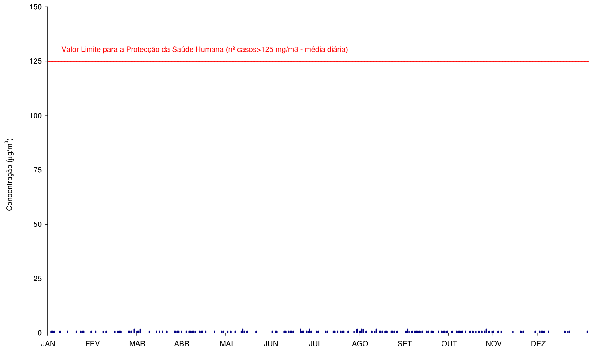
Gráfico 10 - Médias diárias das concentrações de \text{SO}_2 ( \mu\text{g}/\text{m}^3 ) registadas em Salgueiro (Janeiro a Dezembro de 2011).
