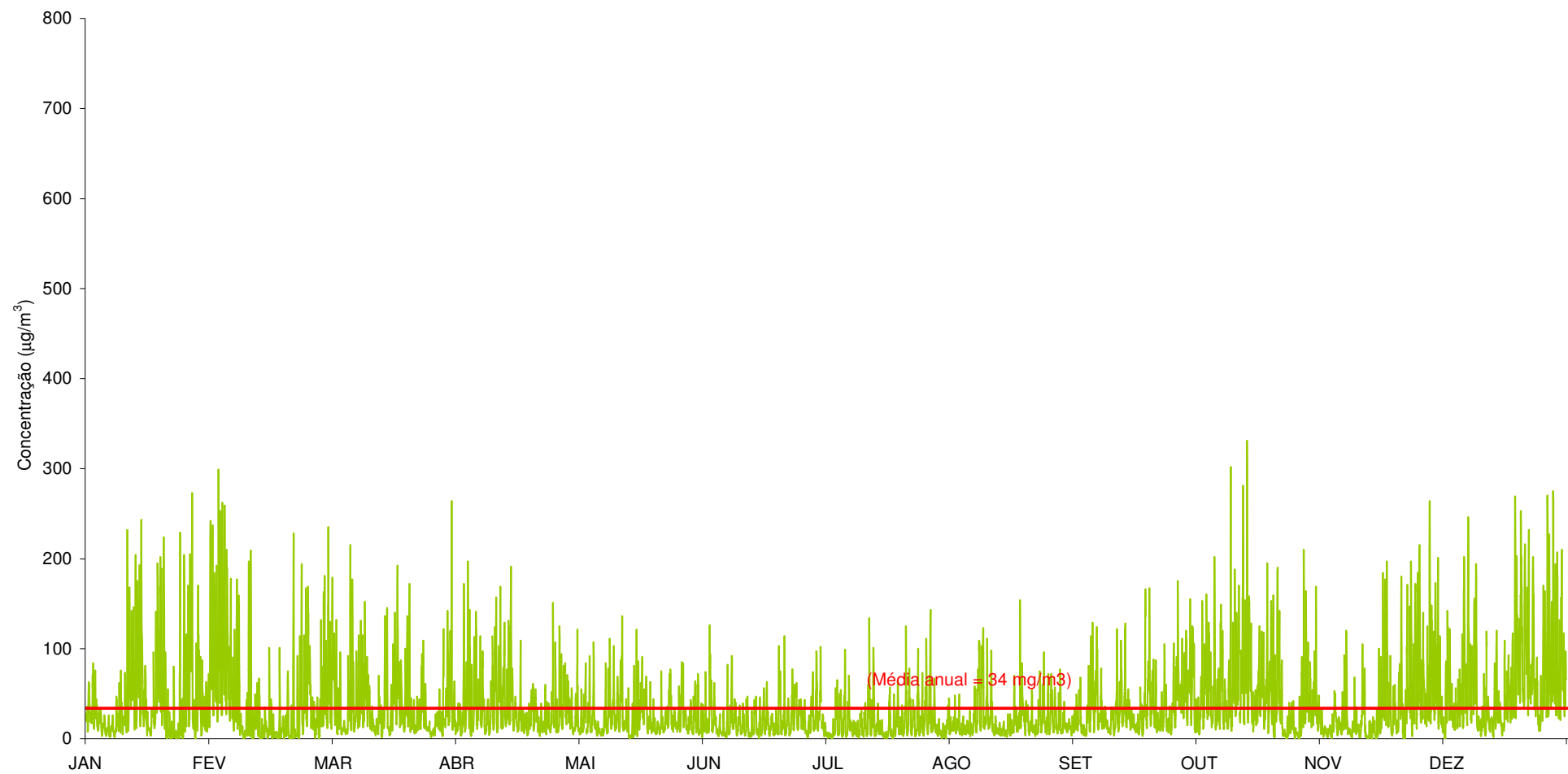
Gráfico 36 - Médias horárias das concentrações de \text{NO}_x ( \mu\text{g}/\text{m}^3 ) registadas na Teixugueira (Janeiro a Dezembro de 2011).
