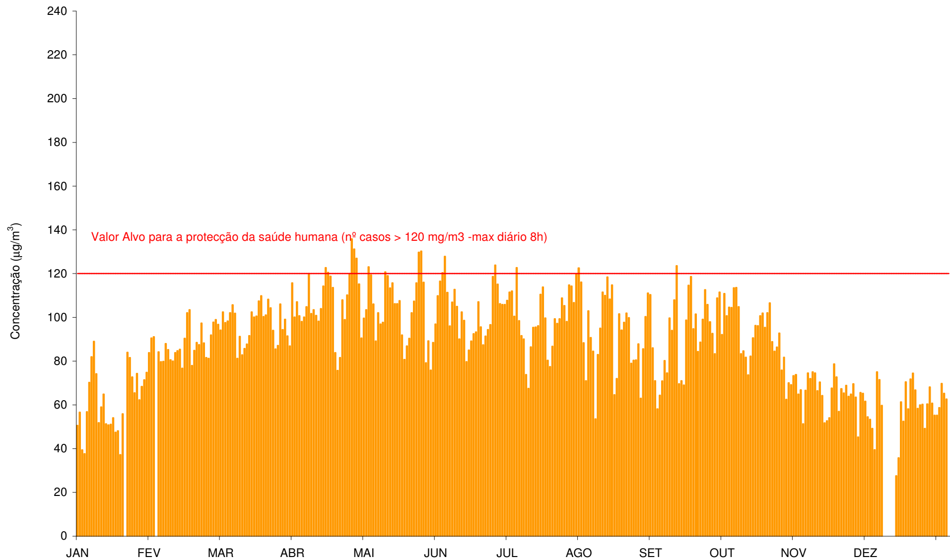
Gráfico 50 - Máximo das médias octo-horárias do dia das concentrações de \text{O}_3 ( \mu\text{g}/\text{m}^3 ) registadas em Salgueiro (Janeiro a Dezembro de 2011).
