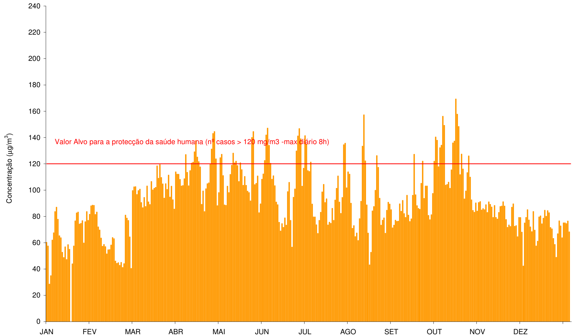
Gráfico 53 - Máximo das médias octo-horárias do dia das concentrações de O 3 ( \mu\text{g}/\text{m}^3 ) registadas em Montemor-o-Velho (Janeiro a Dezembro de 2011).
