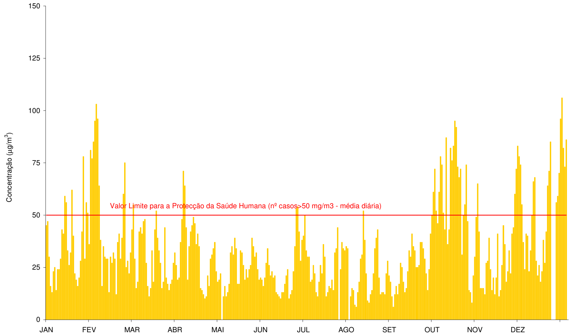
Gráfico 74 – Médias diárias das concentrações de PM10 ( \mu\text{g}/\text{m}^3 ) registadas na Teixugueira (Janeiro a Dezembro de 2011).
