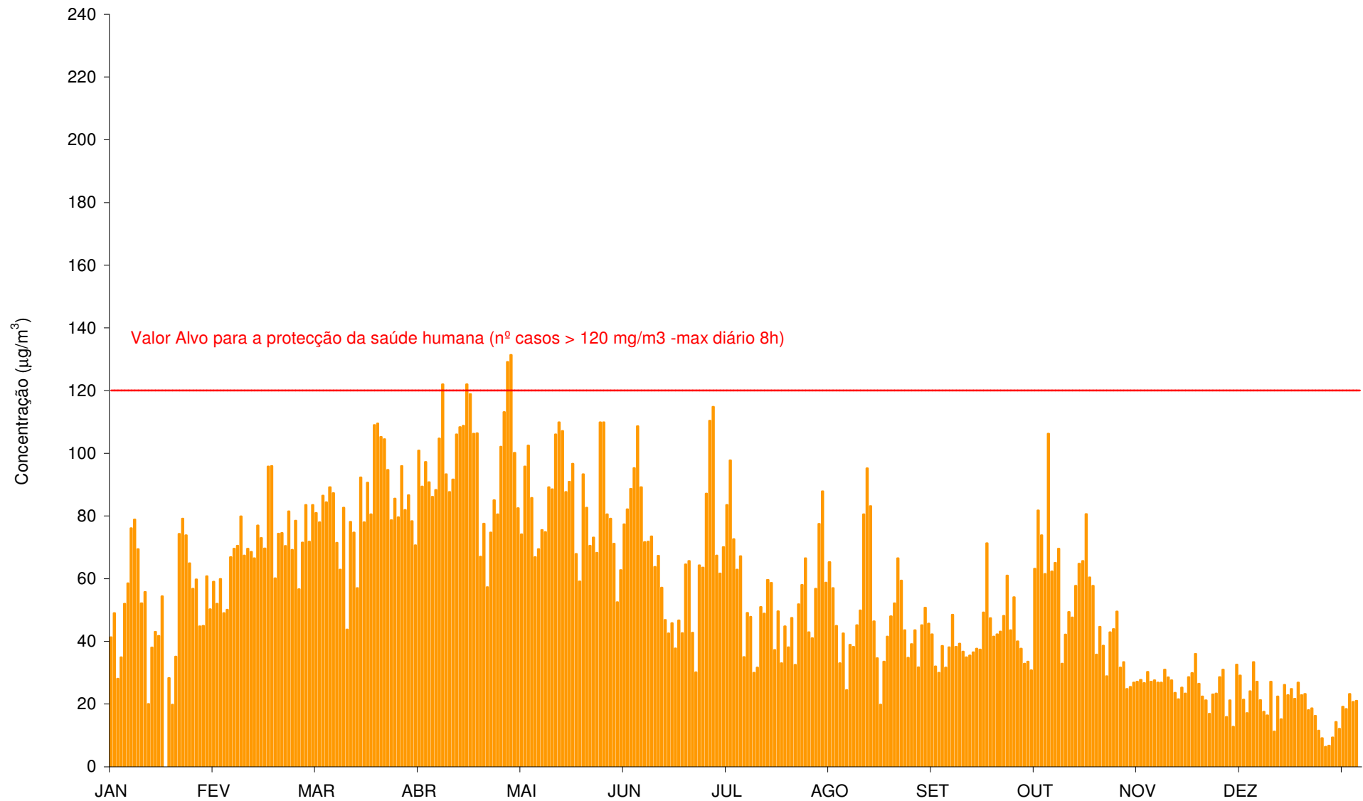
Gráfico 54 - Máximo das médias octo-horárias do dia das concentrações de O 3 ( \mu\text{g}/\text{m}^3 ) registadas na Teixugueira (Janeiro a Dezembro de 2011).
