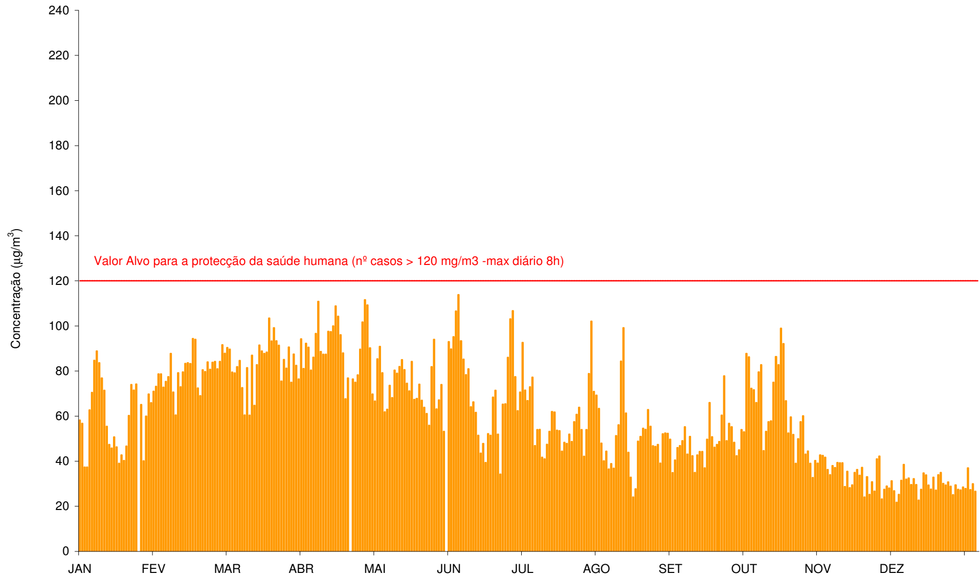
Gráfico 52 - Máximo das médias octo-horárias do dia das concentrações de O 3 ( \mu\text{g}/\text{m}^3 ) registadas em Ervedeira (Janeiro a Dezembro de 2011).
