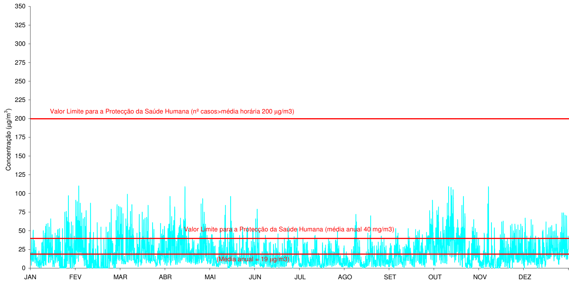
Gráfico 27 - Médias horárias das concentrações de \text{NO}_2 ( \mu\text{g}/\text{m}^3 ) registadas na Teixugueira (Janeiro a Dezembro de 2011).
