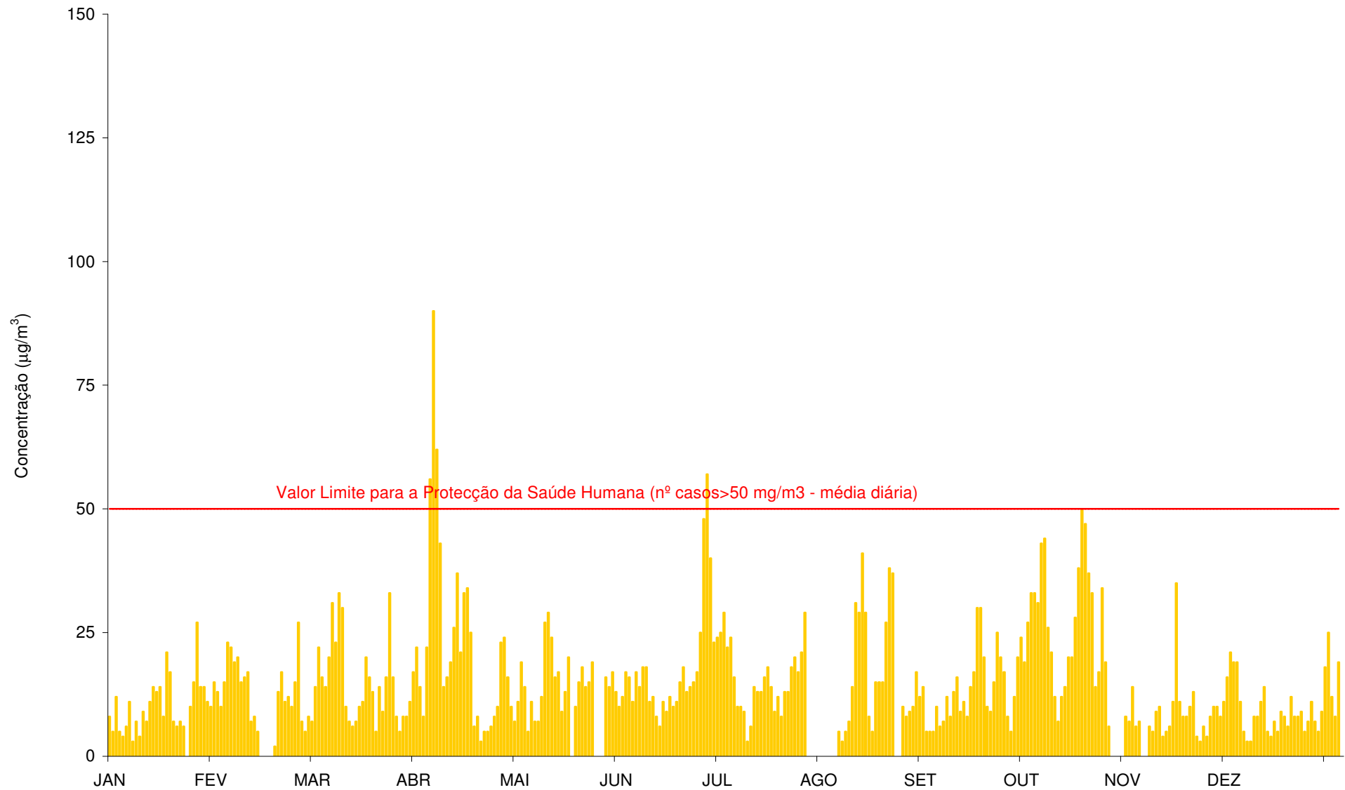
Gráfico 70 – Médias diárias das concentrações de PM10 ( \mu\text{g}/\text{m}^3 ) registadas em Forno do Monte (Janeiro a Dezembro de 2011).
