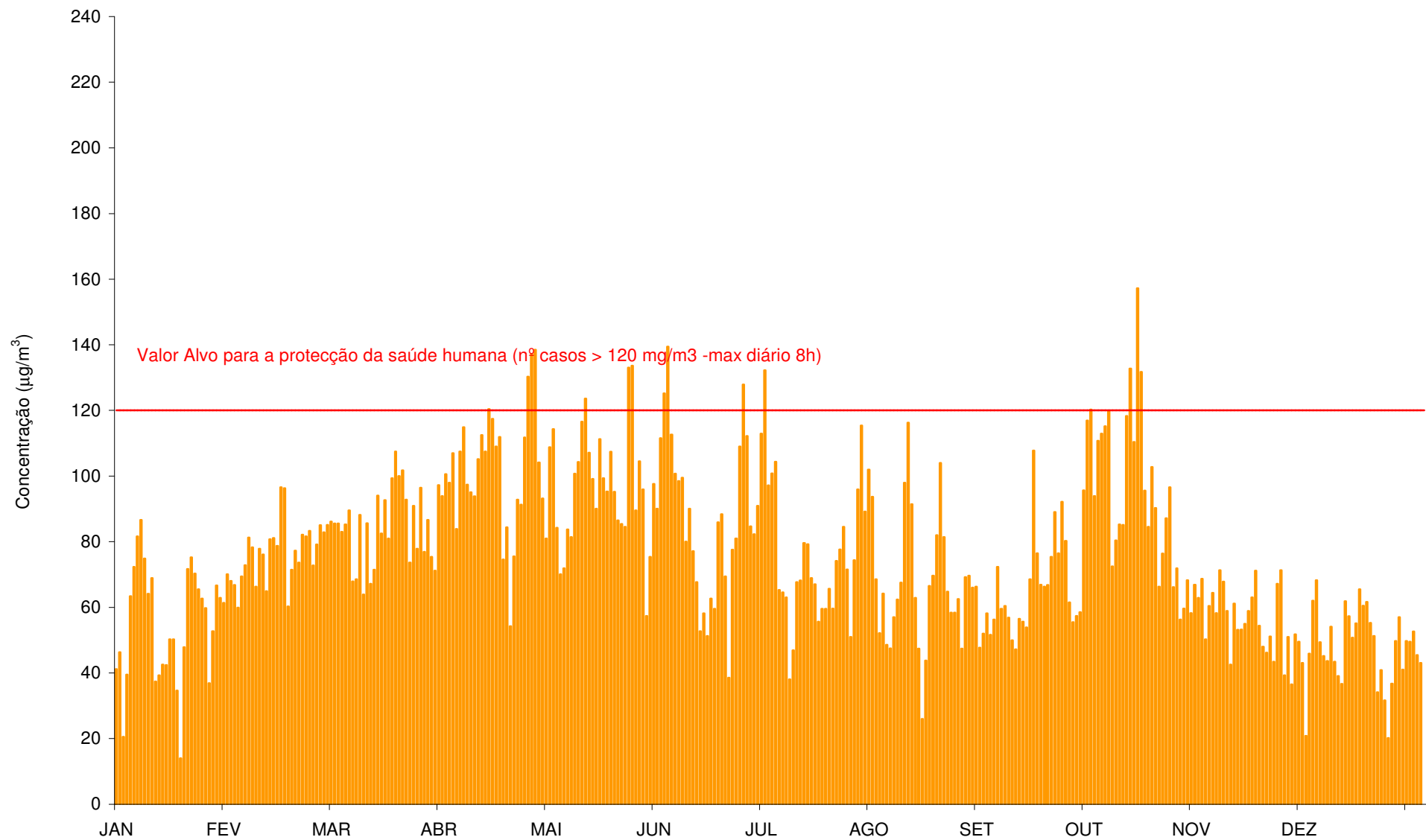
Gráfico 48 - Máximo das médias octo-horárias do dia das concentrações de O 3 ( \mu\text{g}/\text{m}^3 ) registadas em Ílhavo (Janeiro a Dezembro de 2011).
