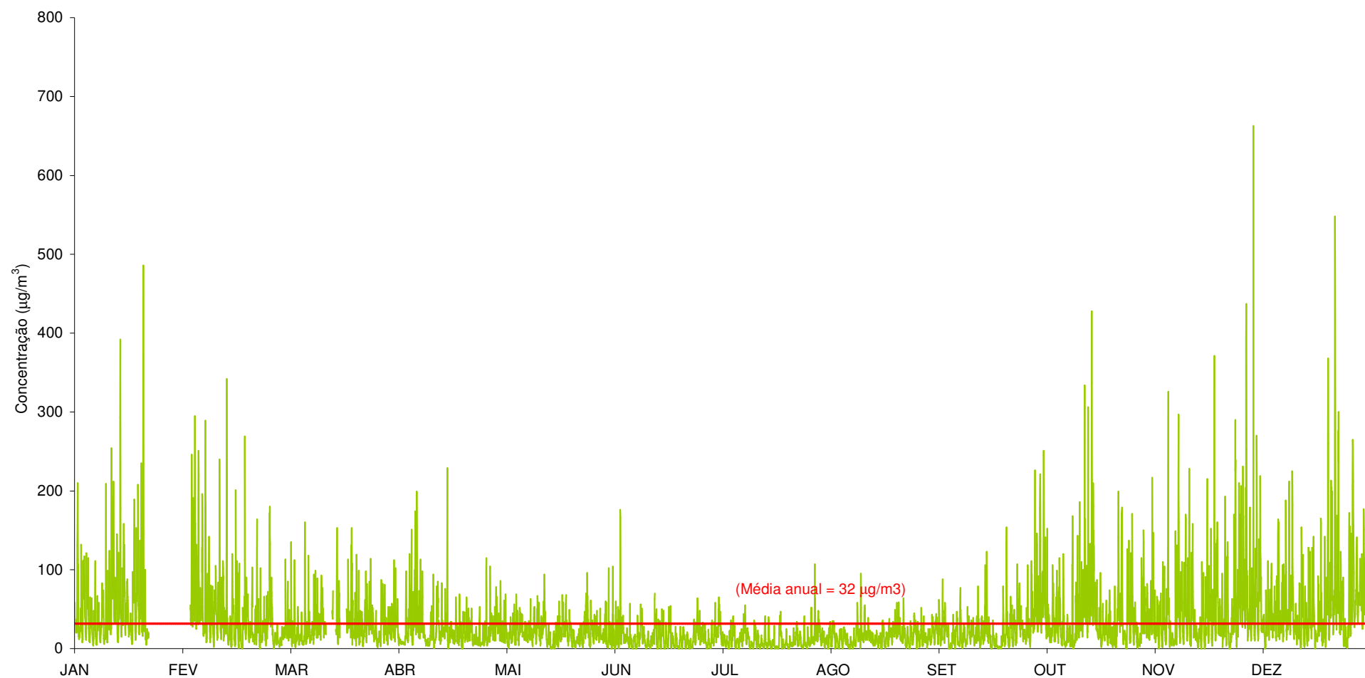
Gráfico 29 - Médias horárias das concentrações de NO x (µg/m 3 ) registadas em Aveiro (Janeiro a Dezembro de 2011).
