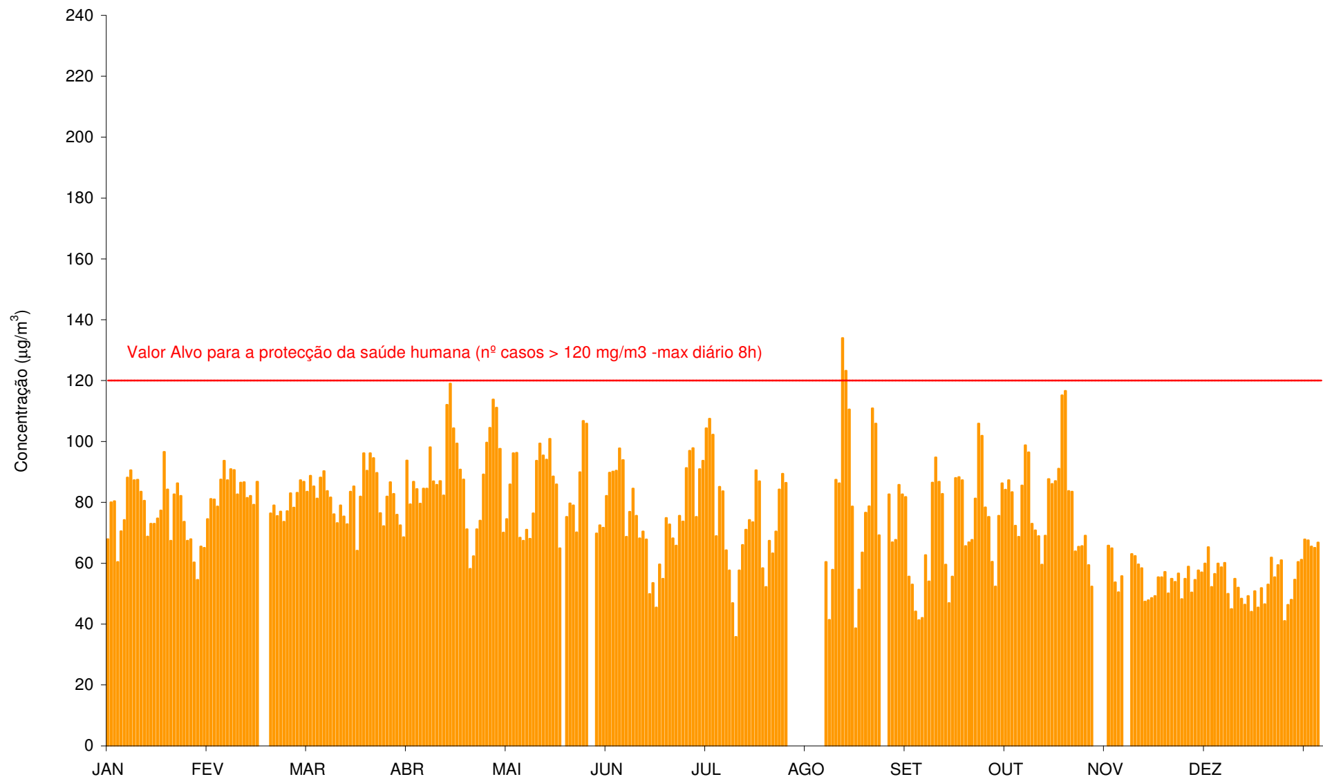
Gráfico 51 - Máximo das médias octo-horárias do dia das concentrações de O 3 ( \mu\text{g}/\text{m}^3 ) registadas em Furnelo do Monte (Janeiro a Dezembro de 2011).
