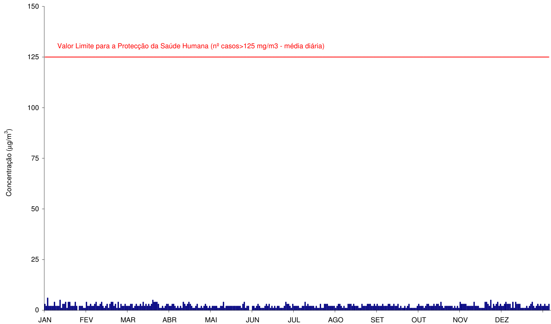
Gráfico 12 - Médias diárias das concentrações de SO 2 (µg/m 3 ) registadas em Ervedeira (Janeiro a Dezembro de 2011).
