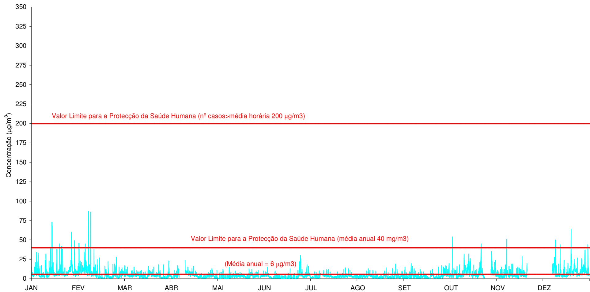
Gráfico 24 - Médias horárias das concentrações de \text{NO}_2 ( \mu\text{g}/\text{m}^3 ) registadas na Ervedeira (Janeiro a Dezembro de 2011).
