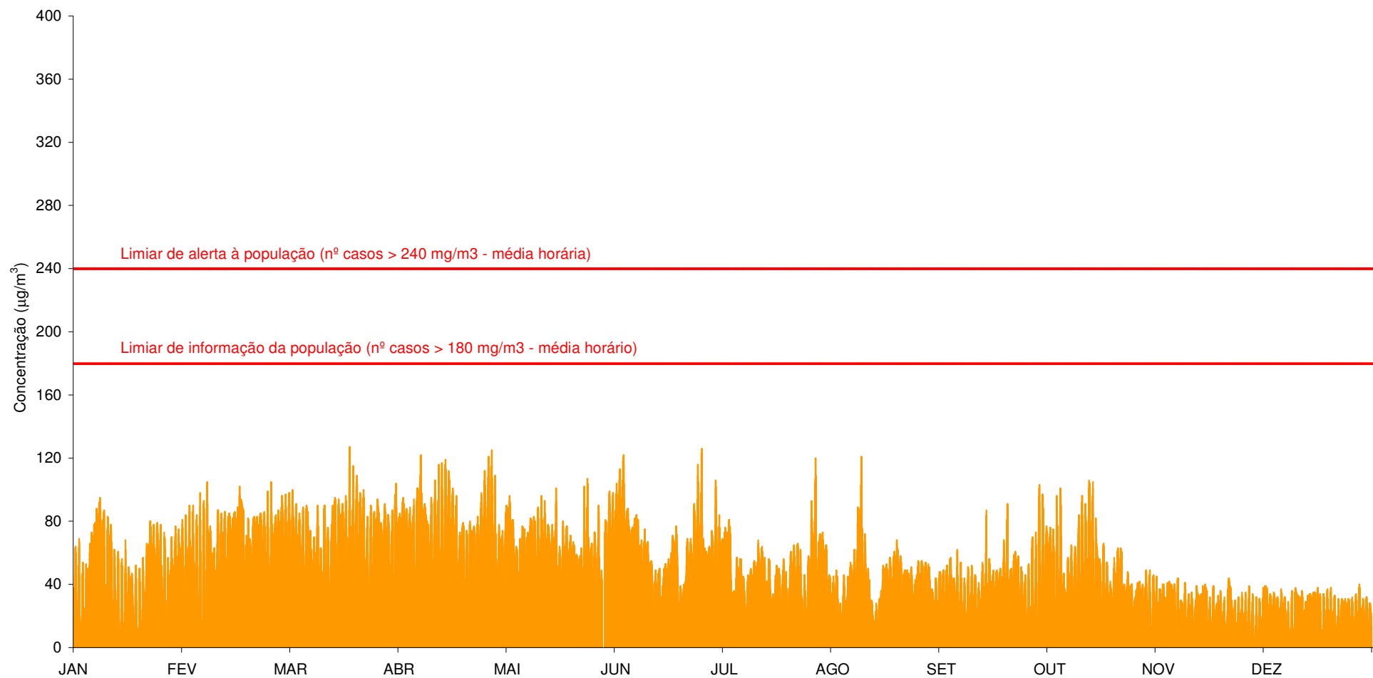
Gráfico 45 - Médias horárias das concentrações de O 3 (µg/m 3 ) registadas em Ervedeira (Janeiro a Dezembro de 2011).
