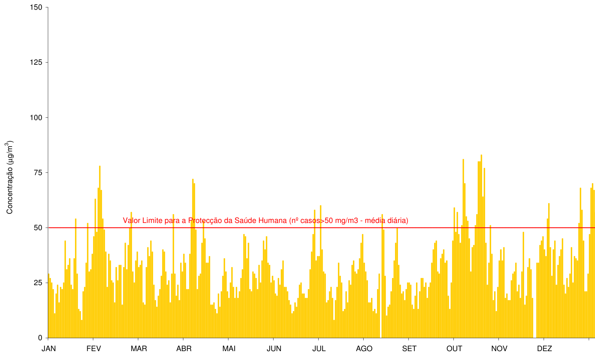
Gráfico 72 – Médias diárias das concentrações de PM10 ( \mu\text{g}/\text{m}^3 ) registadas na Fernão Magalhães (Janeiro a Dezembro de 2011).
