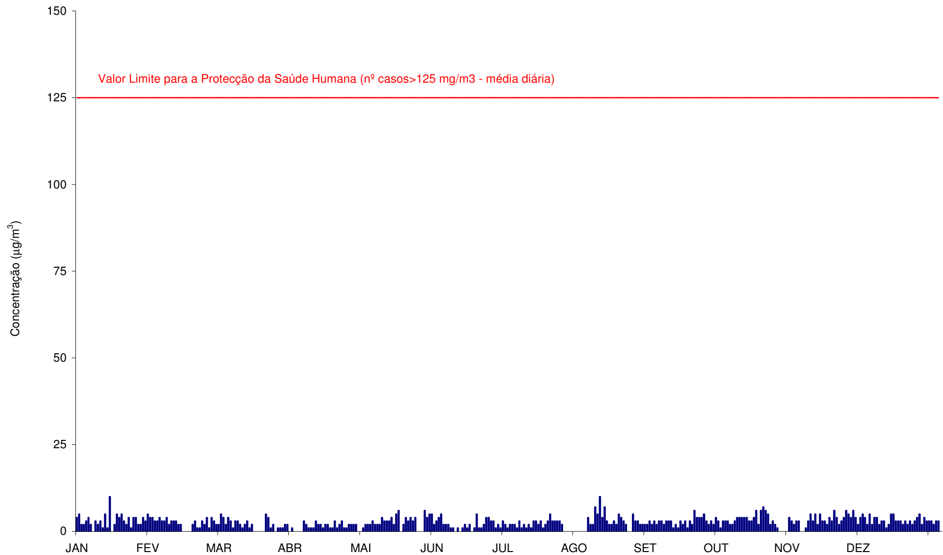
Gráfico 11 - Médias diárias das concentrações de SO 2 (µg/m 3 ) registadas em Forno do Monte (Janeiro a Dezembro de 2011).
