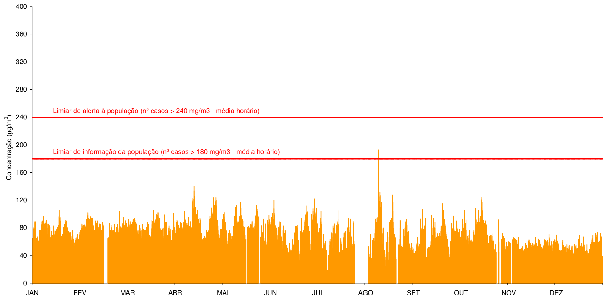
Gráfico 44 - Médias horárias das concentrações de O 3 (µg/m 3 ) registadas em Forno do Monte (Janeiro a Dezembro de 2011).
