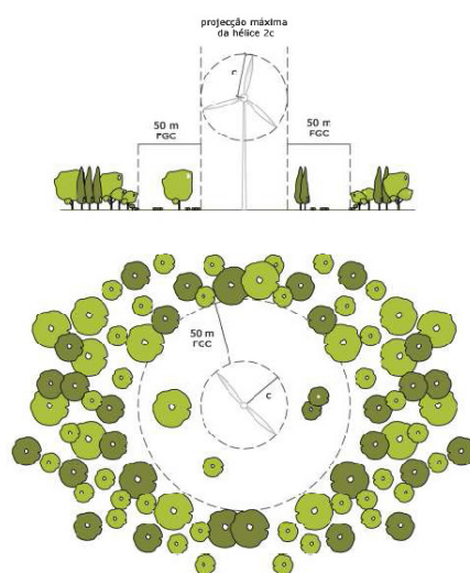
Esquema de faixa de gestão de combustível em aerogerador
